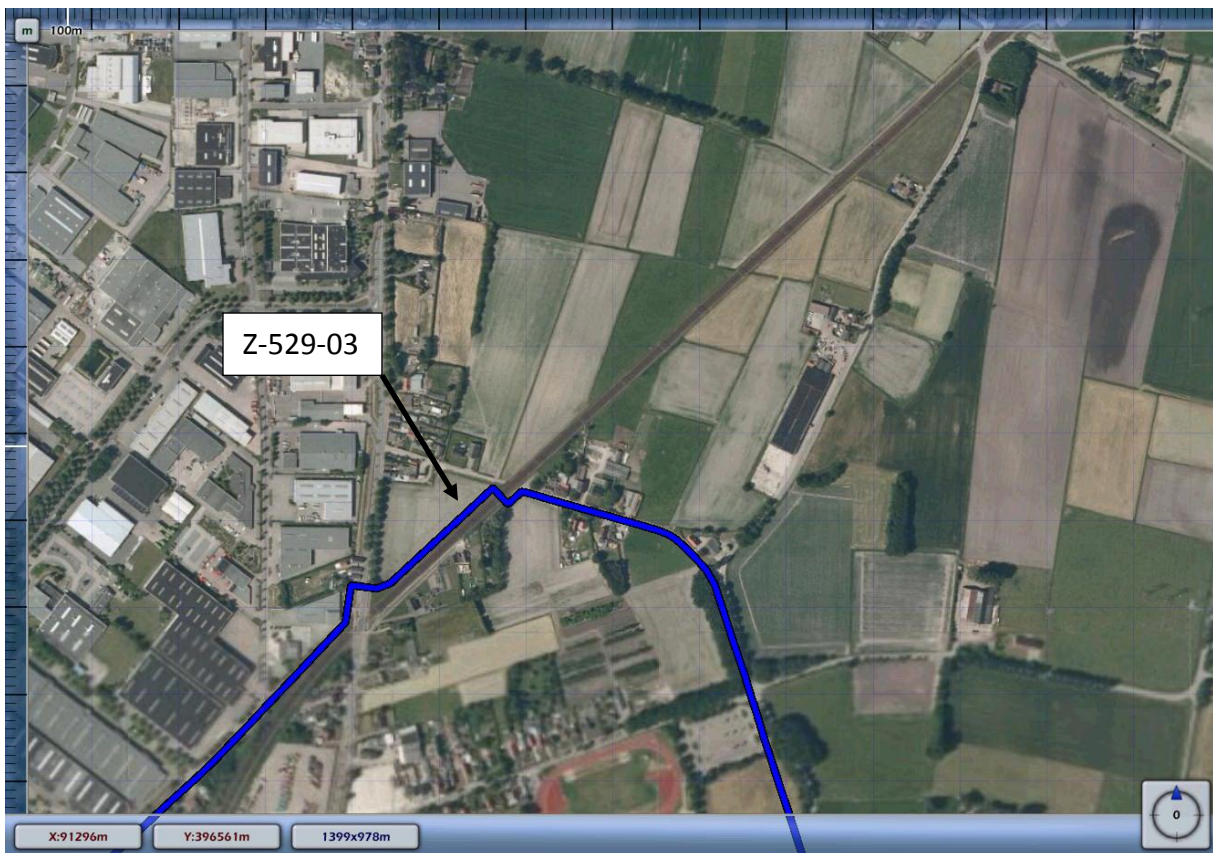
Figuur : Geografische ligging hogedruk aardgasleidingen
