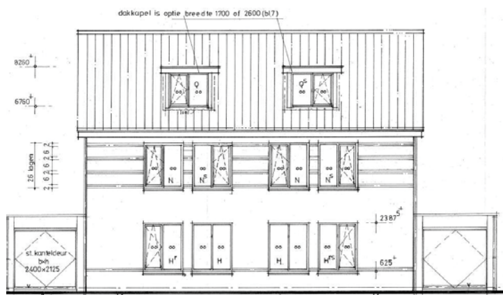
Voorgevel
