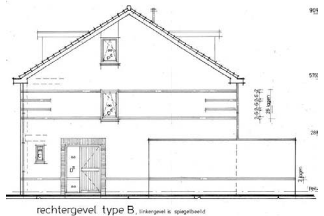
Rechter zijgevel
