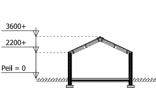
doorsnede gebouw 5
