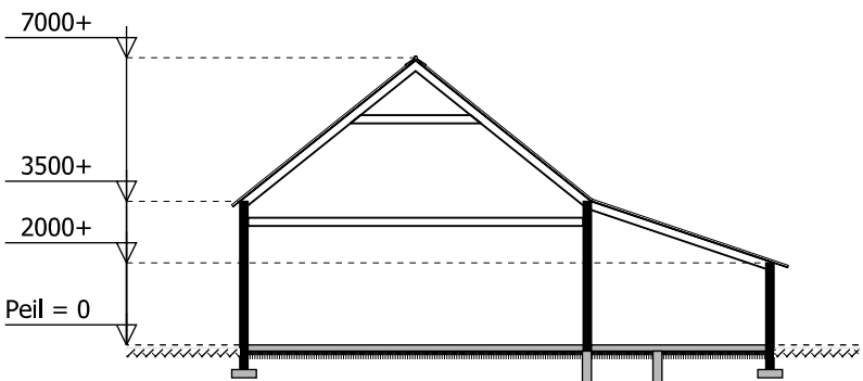
doorsnede gebouw 2
