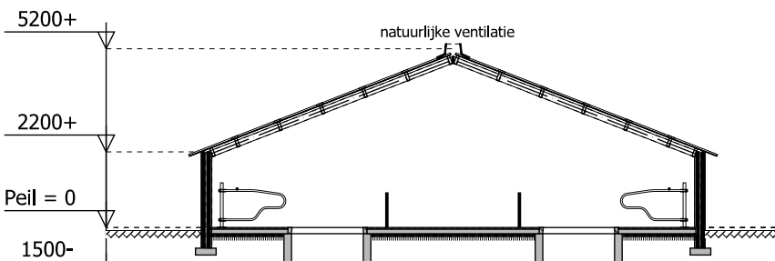
doorsnede gebouw 3
