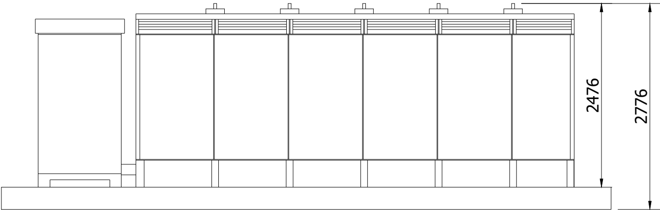
Vooraanzicht
