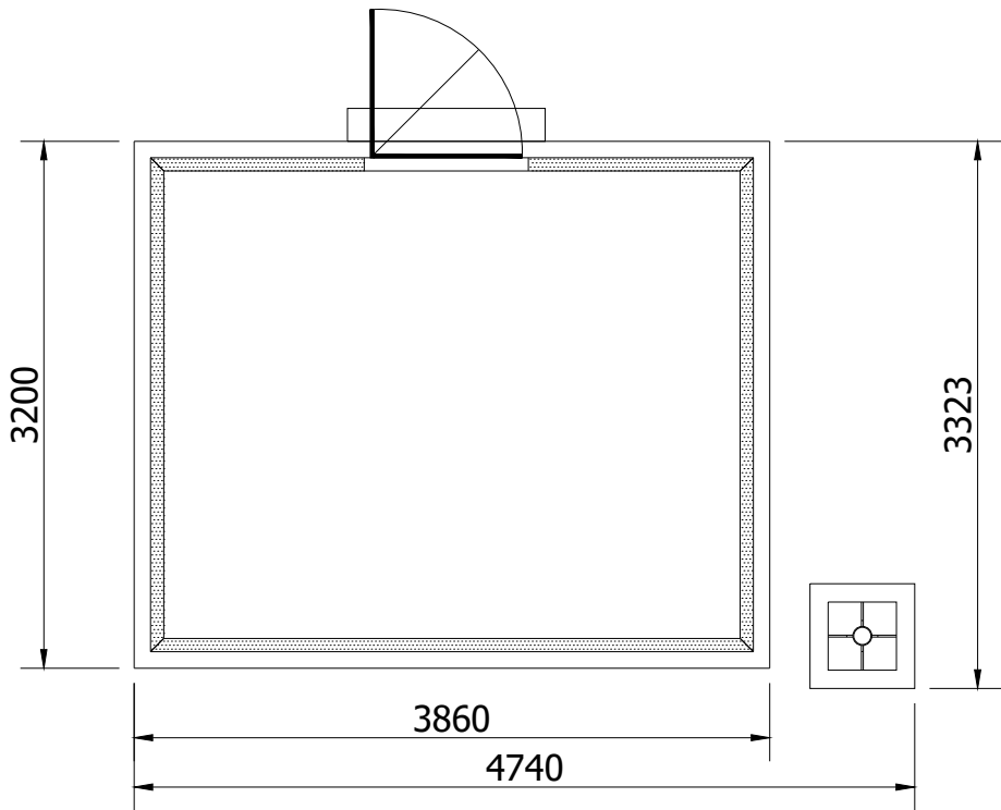
PLATTEGROND
