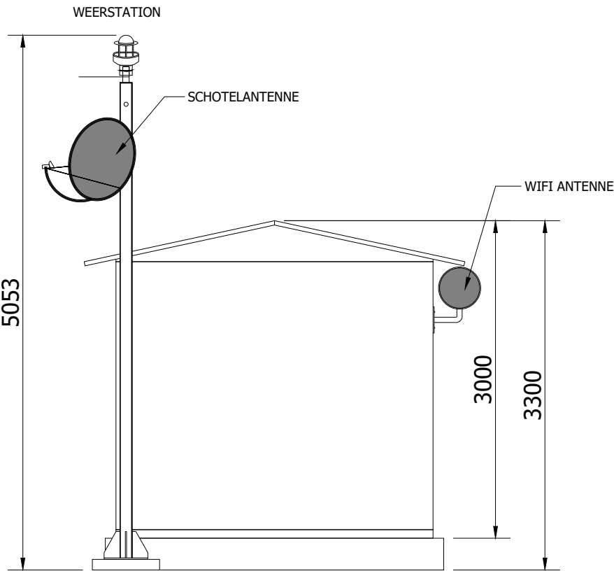
ZIJAAANZICHT
