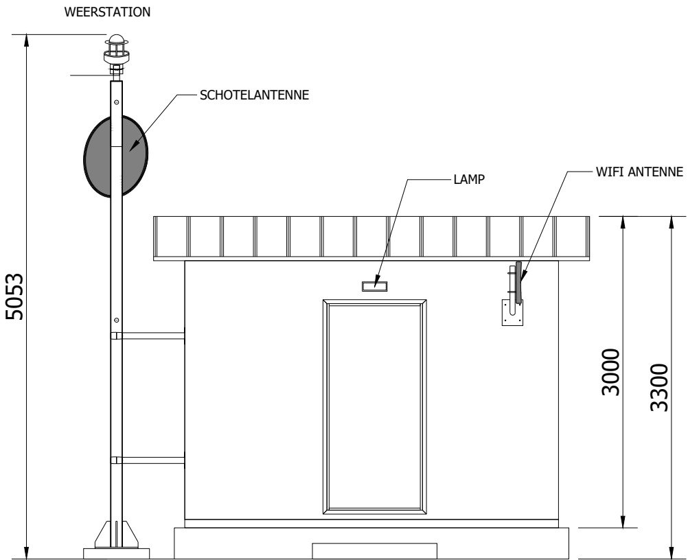
VOORAANZICHT
