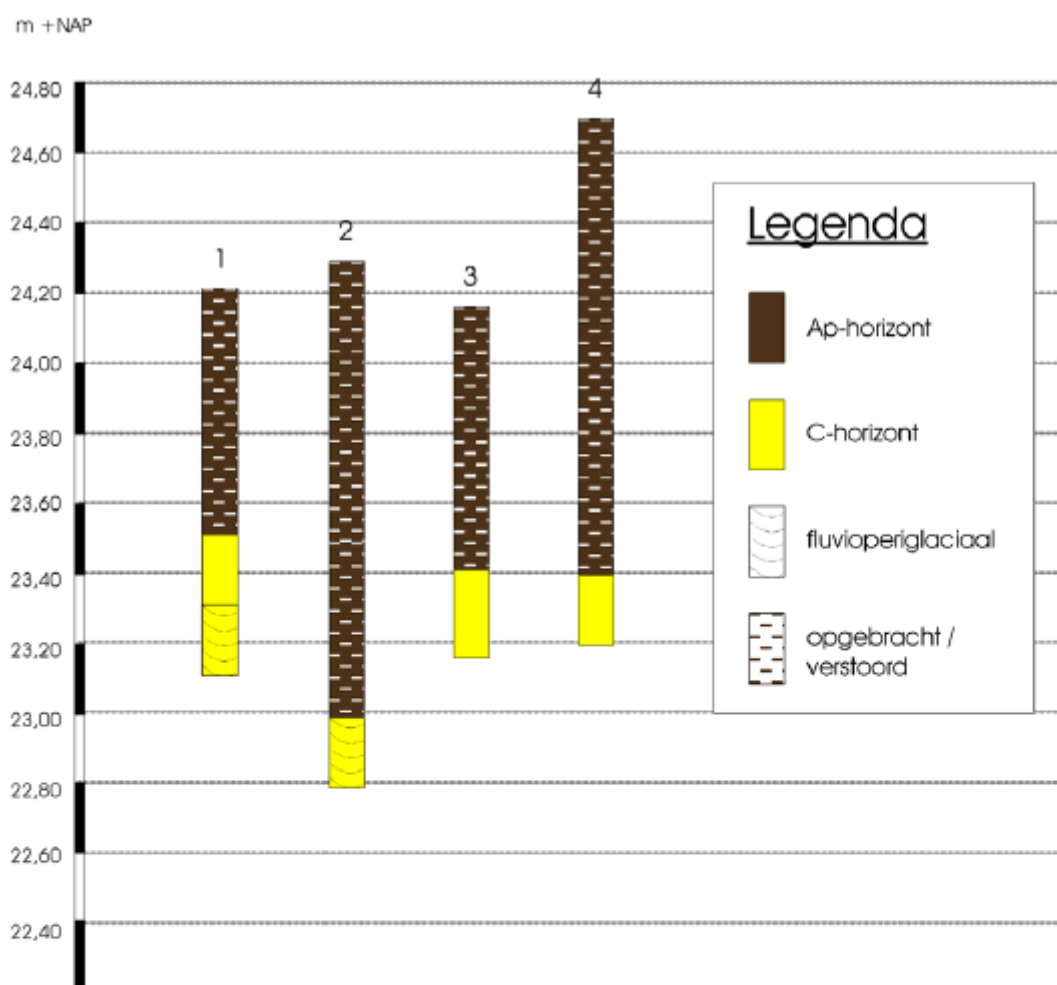
Figuur 10: Boorprofielen
