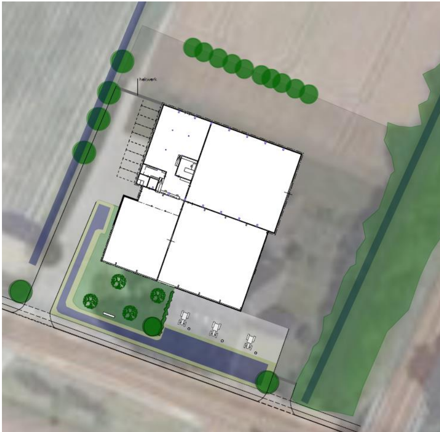
Schetsontwerp toekomstige situatie (bron: Ontwerpstation Loppersum)
