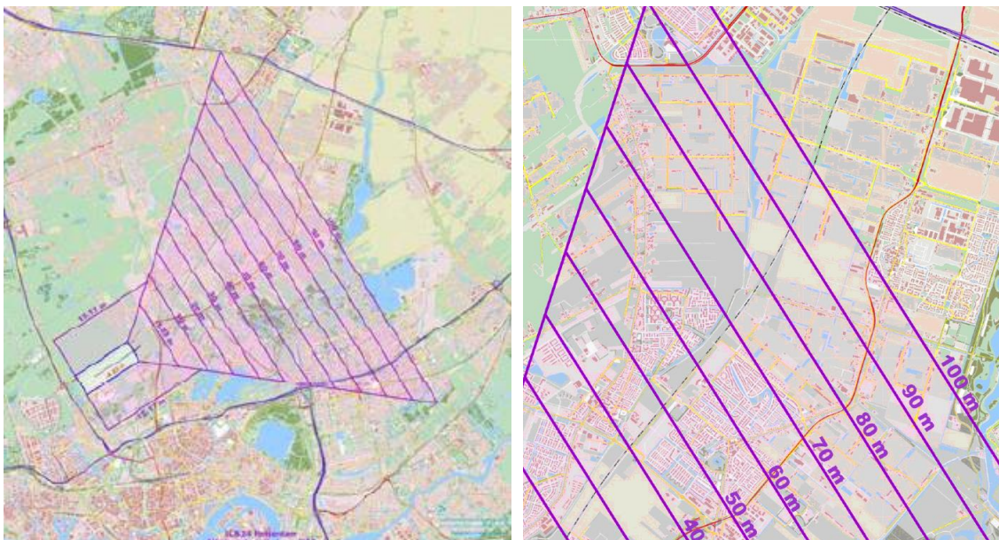
Afbeelding 7.3: toetsingsvlakken ILS 24
