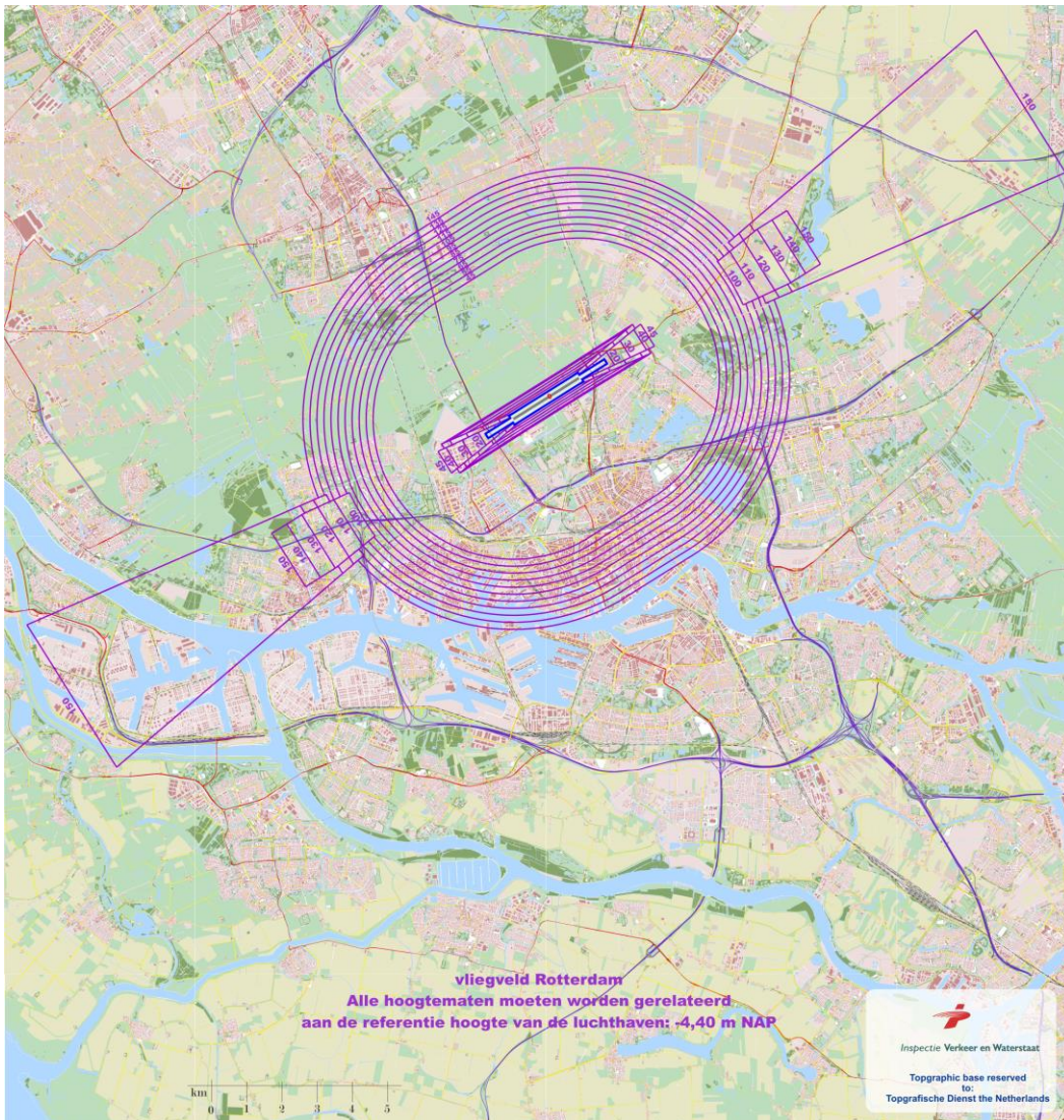
Afbeelding7.5: Hoogtebeperking invliegfunnel
