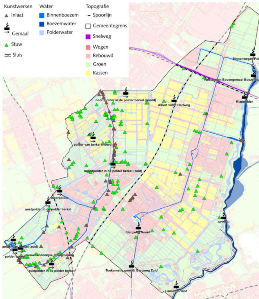
Afbeelding 5.1: watersysteem Lansingerland
