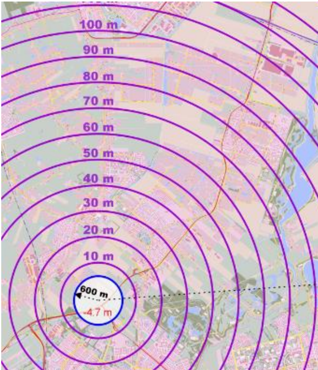
Afbeelding 7.4: Hoogtebeperking DVOR/DME
