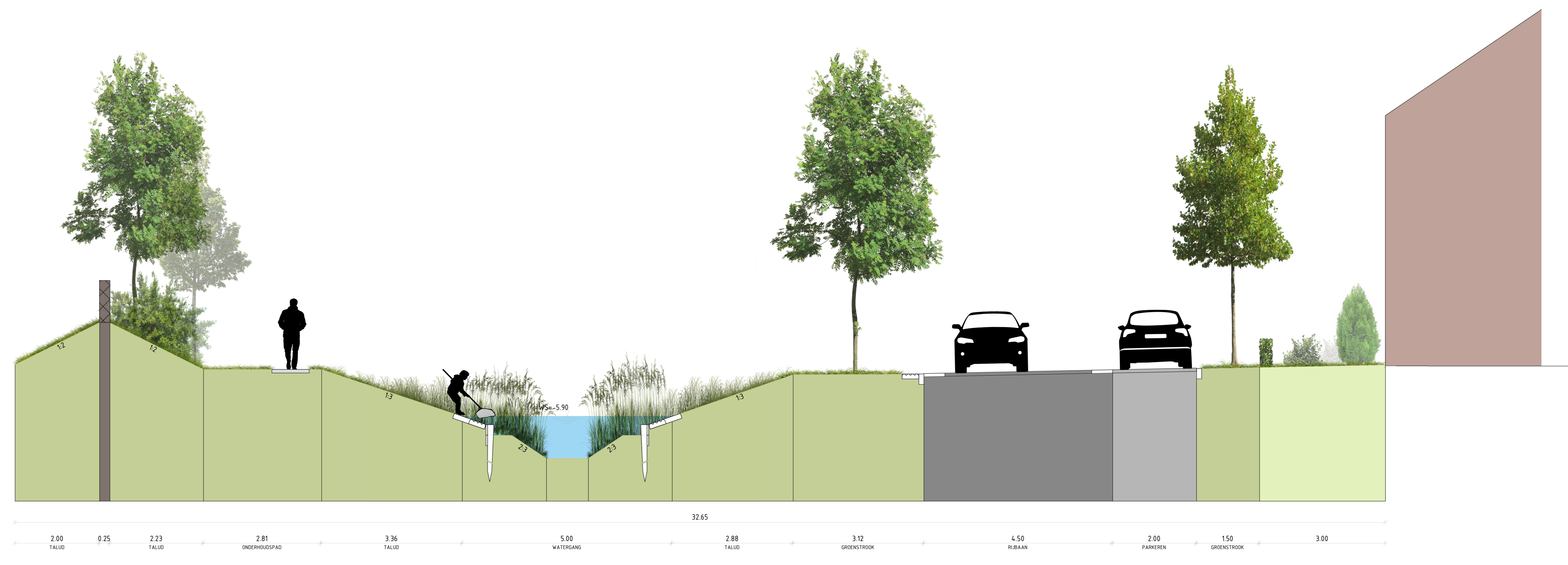
DWARSPROFIEL 5 Woonstraat, langs parkeren met watergang
