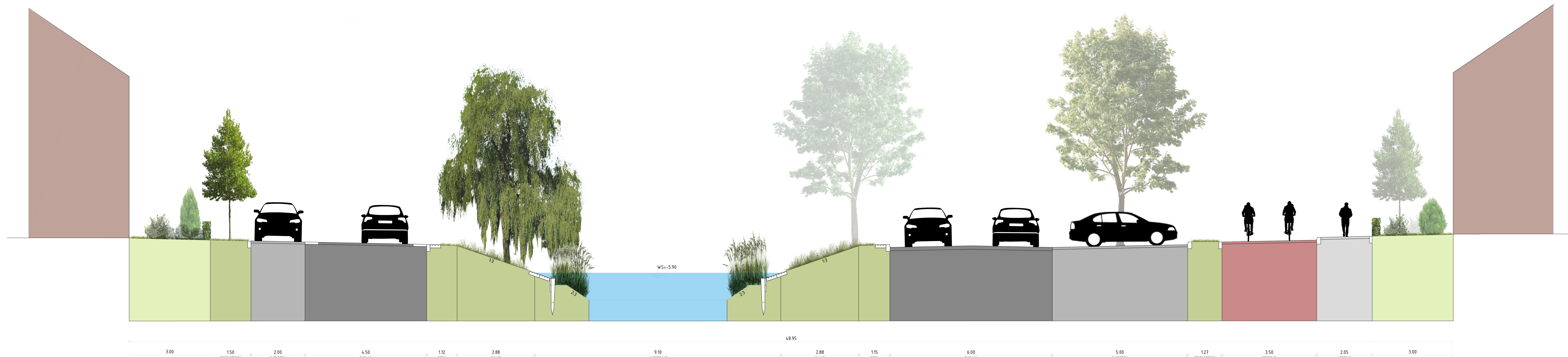
DWARSPROFIEL 1 Louis d'Orlaan, watergang en woonstraat
