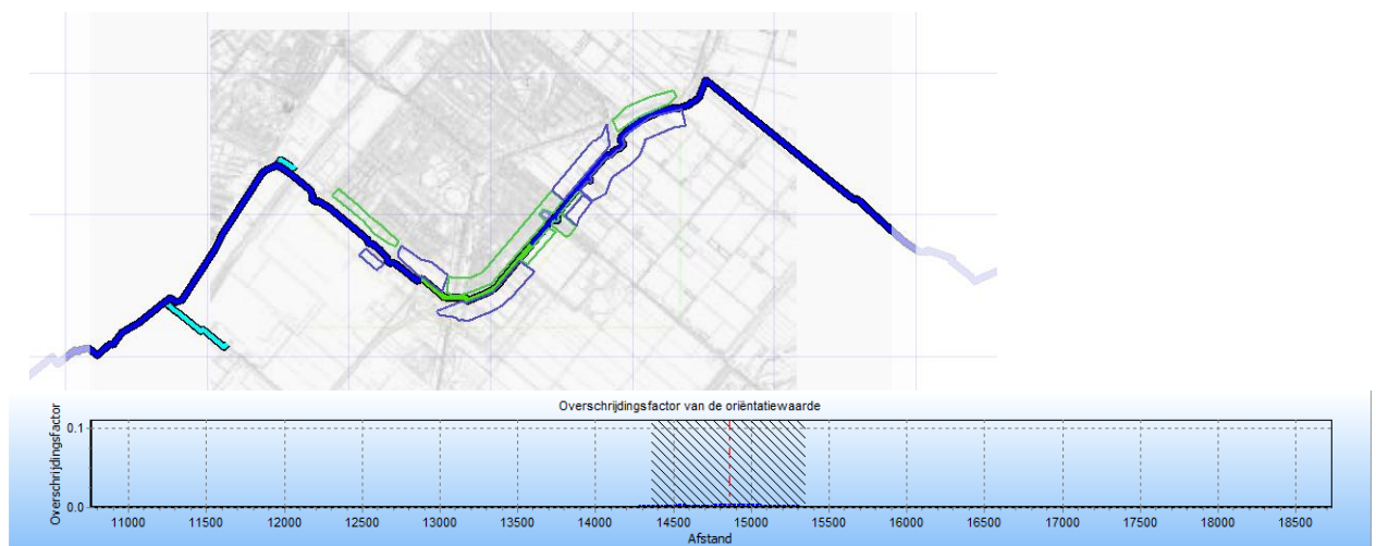
Figuur 4.1 Kilometer met maximale overschrijding van de FN-curve voor W-521-01
