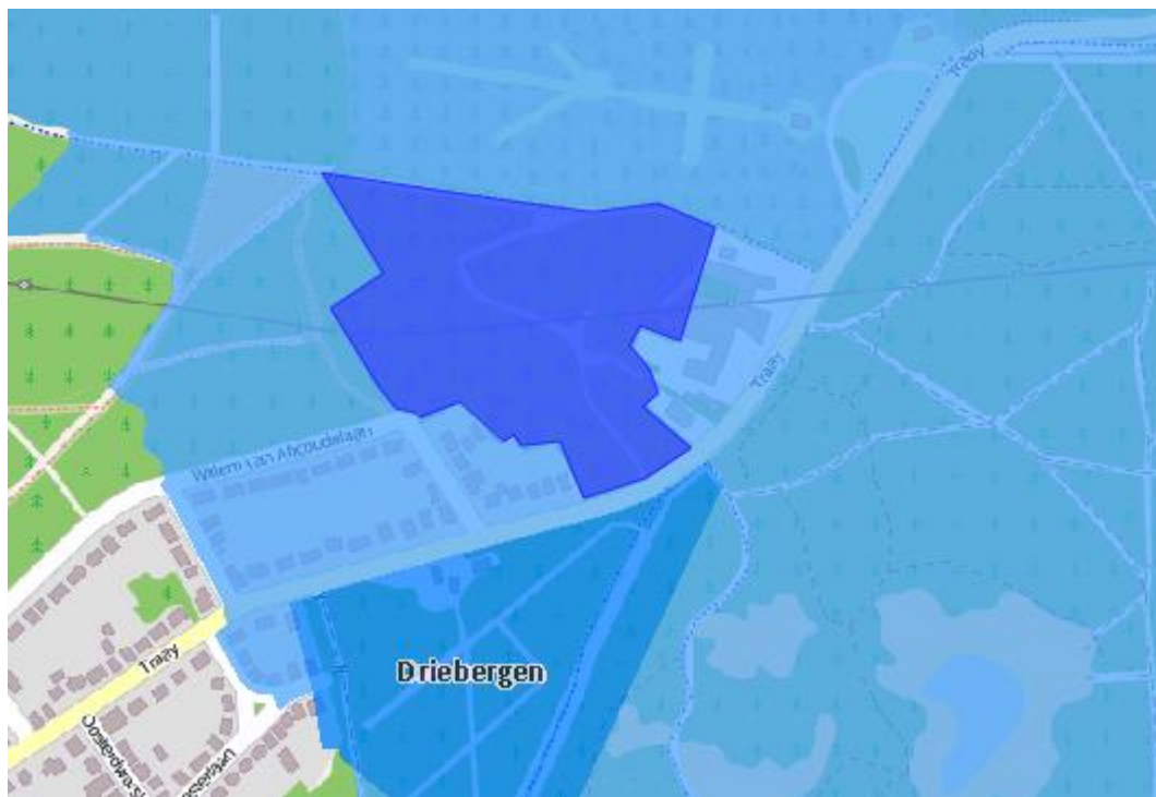
Figuur 2 Ligging recreatieterreinen aan de Willem van Abcoudeaan en de Traaij 299 te Driebergen ten opzichte van het grondwaterbeschermingsgebied Driebergen (lichtblauw). Het waterwinbegebied (donkerblauw) bevindt zich aan de overzijde van de Traaij.
