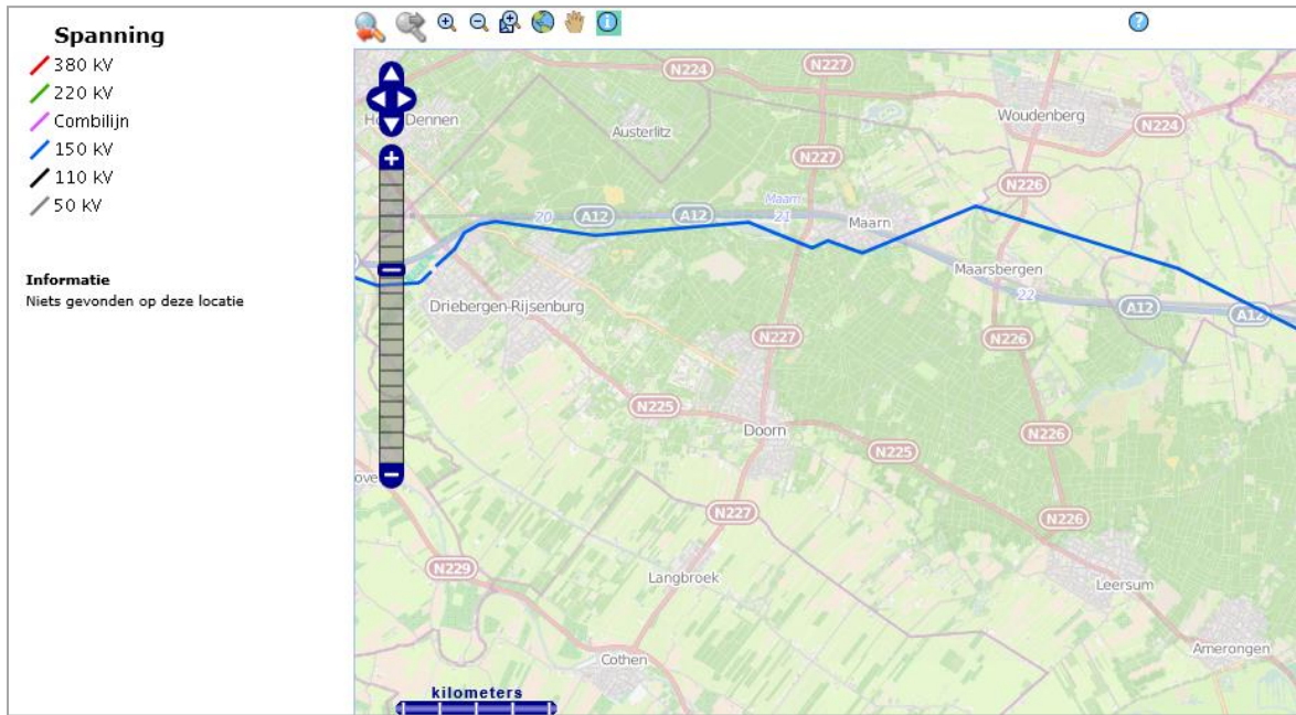
Figuur 7: Hoogspanningslijn (Bron: RIVM/Netkaart HS-lijnen)
