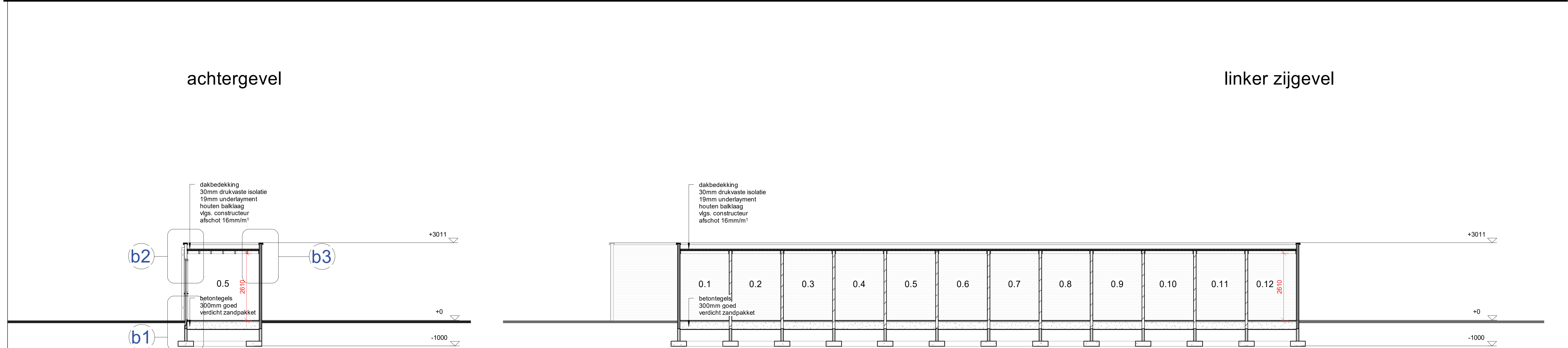
doorsnede A-A
