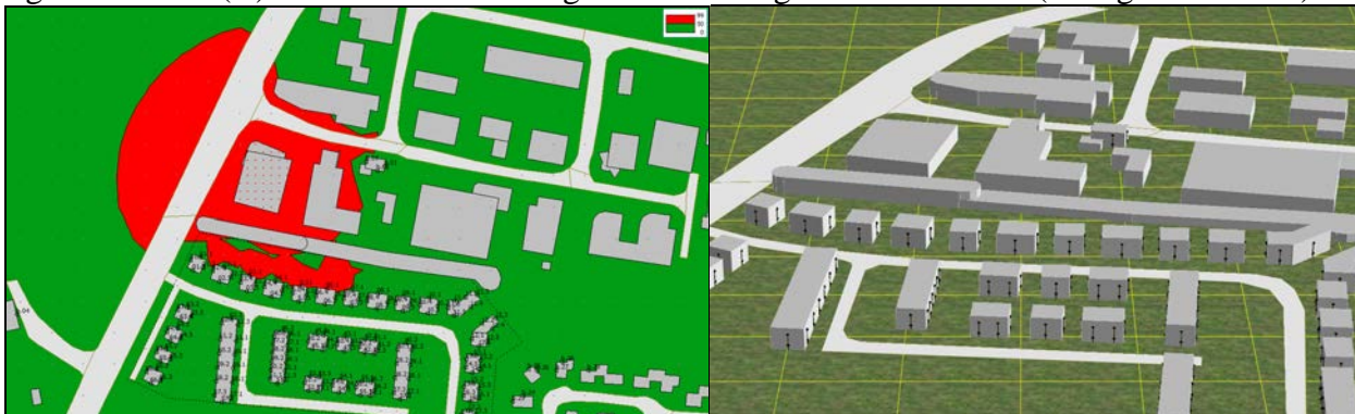
figuur 2: 50 dB(A) contour van fictieve geluiduitstraling milieuklasse 3.2 (incl. grondwal 6m)
