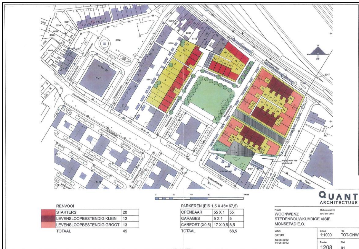
Figuur 3. Plantekening
