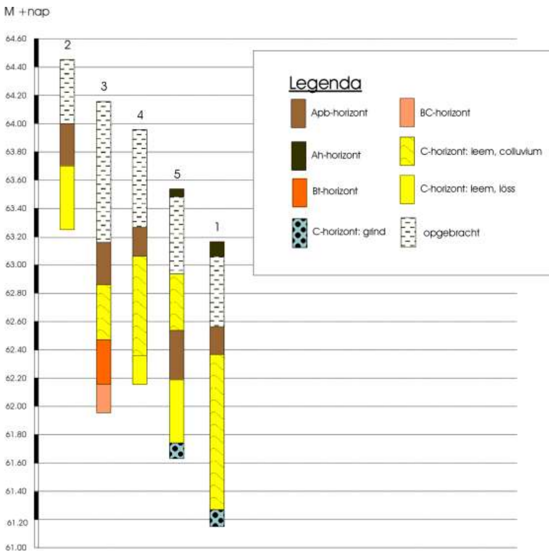
Figuur 24: Boorprofielen
