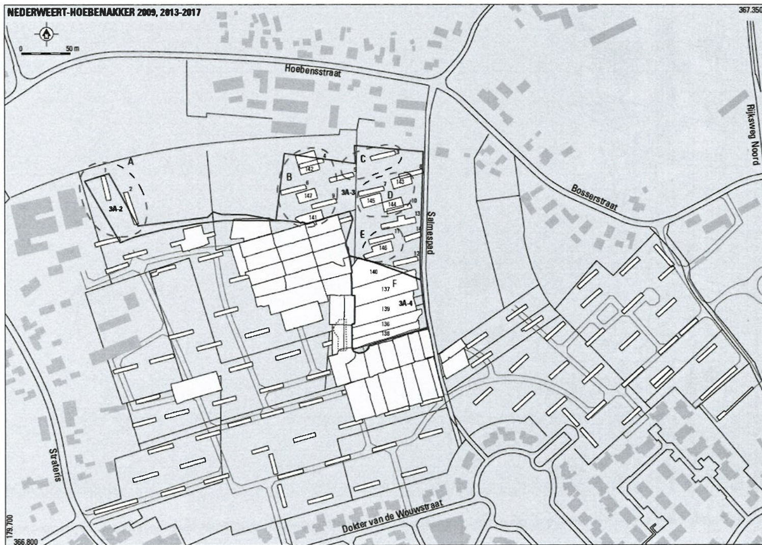
Fig. 1. Nederweert-Hoebenakker. Overzicht van het onderzochte areaal; proefsleuven en werkputten van 2017 in wit met nummers; grens plangebied in blauw; zones met sporen in groen. Schaal 1:3500.
