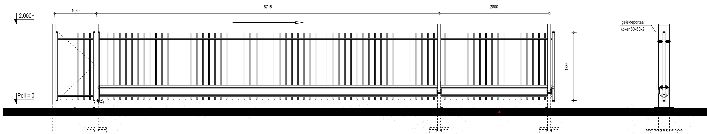
Aanzicht 1
