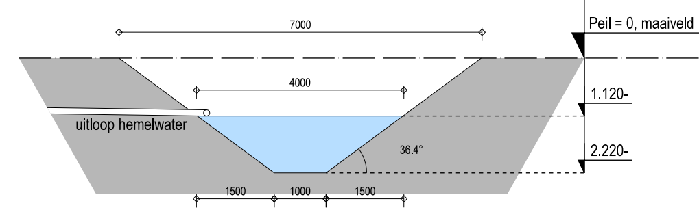
Doorsnede Wadi
