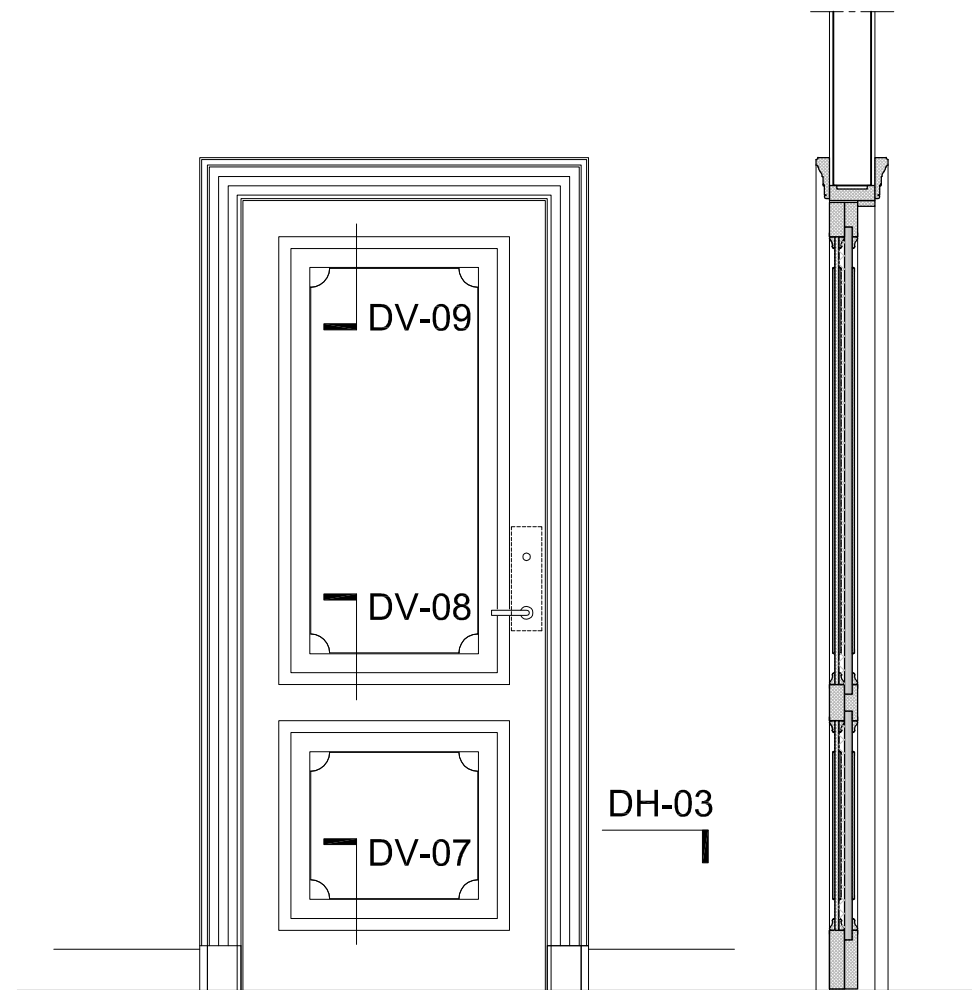
Paneeldeur type A
