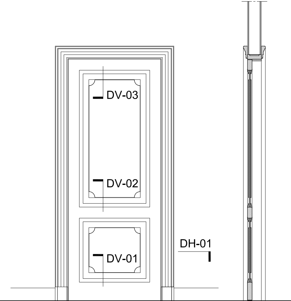
Paneeldeur type A
