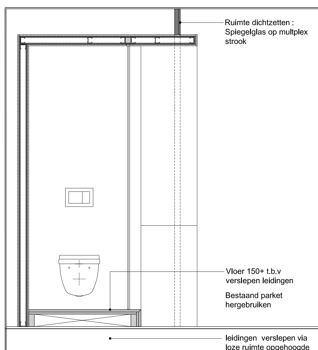
Doorsnede A
