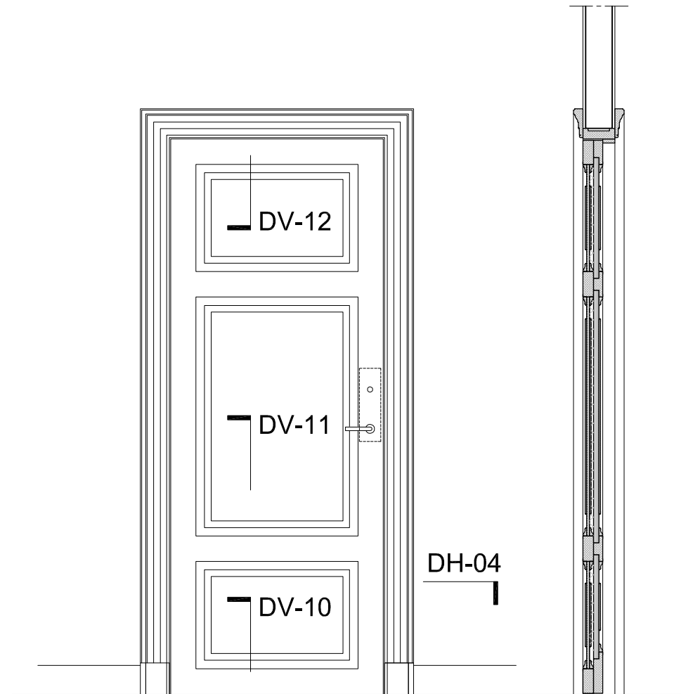
Paneeldeur type B
