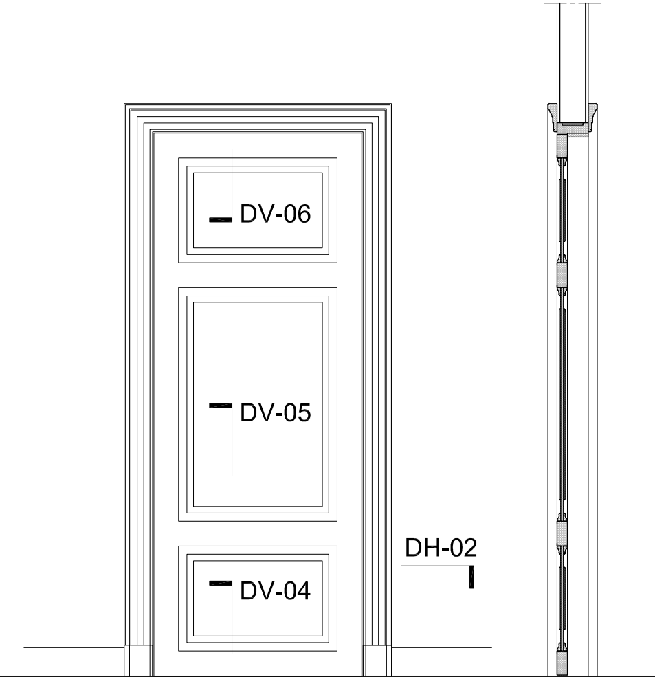
Paneeleur type B
