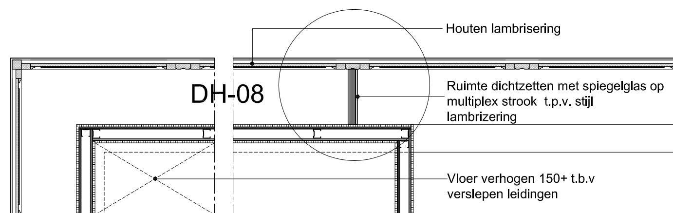
Doorsnede B
