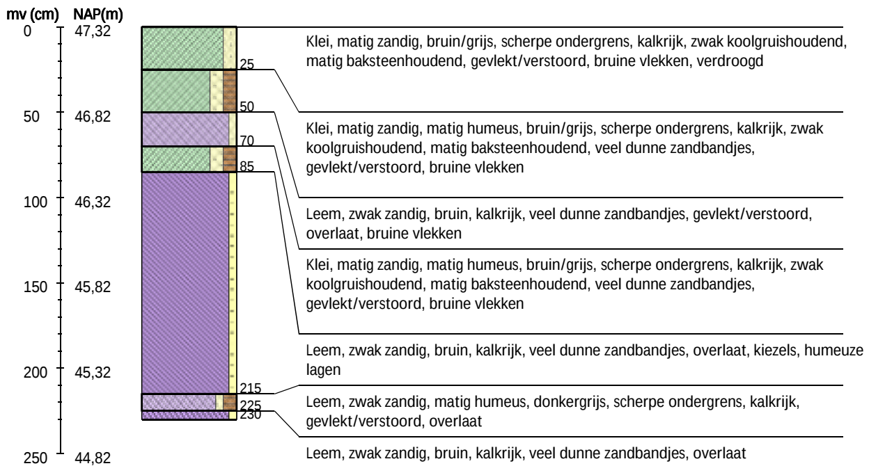
Boring 8 RD-coördinaten: 177836/318876
