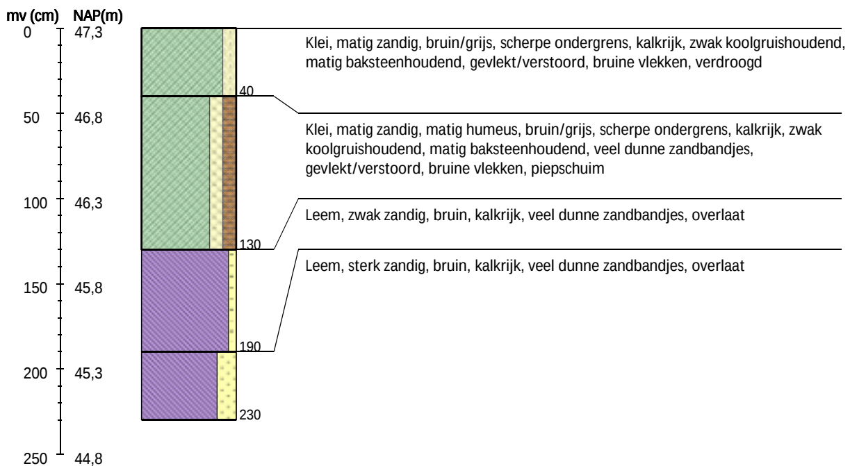
Boring 9 RD-coördinaten: 177855/318868
