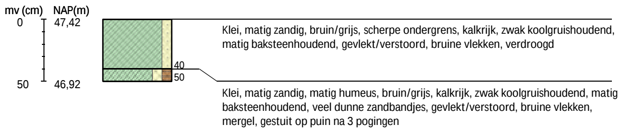
Boring 5 RD-coördinaten: 177763/318909
