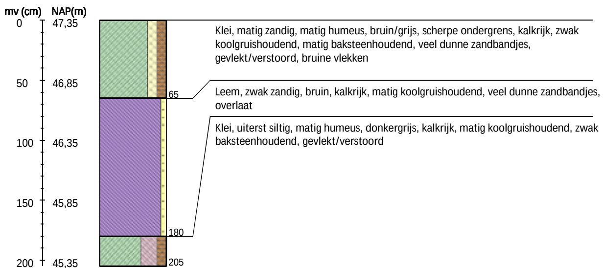
Boring 7 RD-coördinaten: 177807/318889
