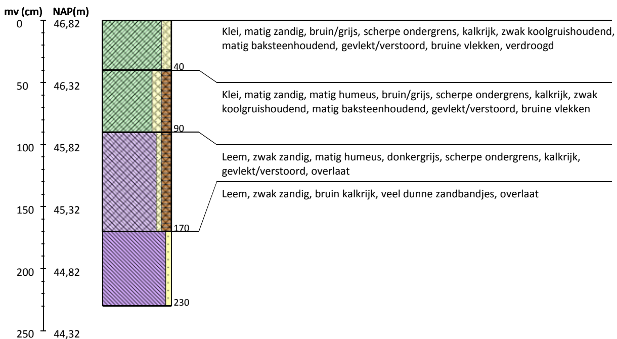
Boring 12 RD-coördinaten: 177927/318860
