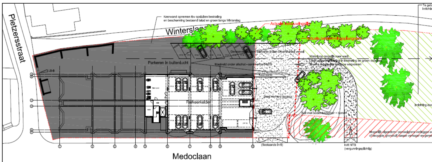
Plattegrond in geval van E-carsharing (10 parkeerplaatsen ten noorden van het gebouw)
