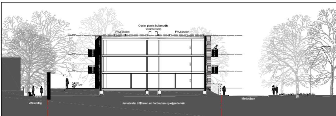
Dwarsdoorsnede van het gebouw
