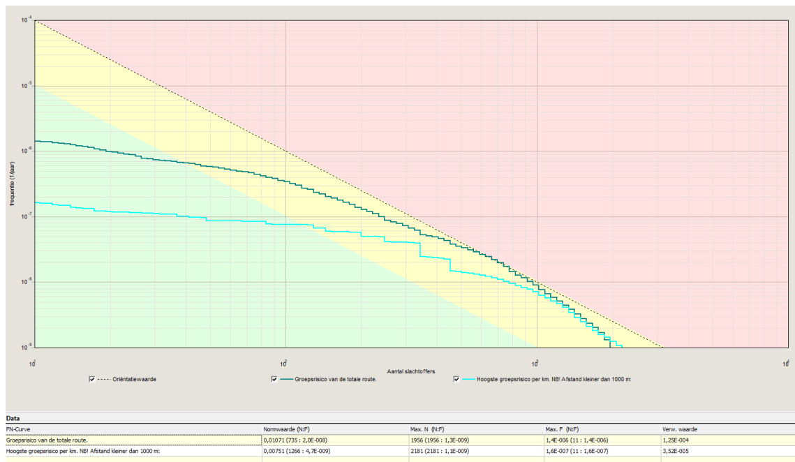
Afbeelding 4 fN-curve berekend groepsrisico
