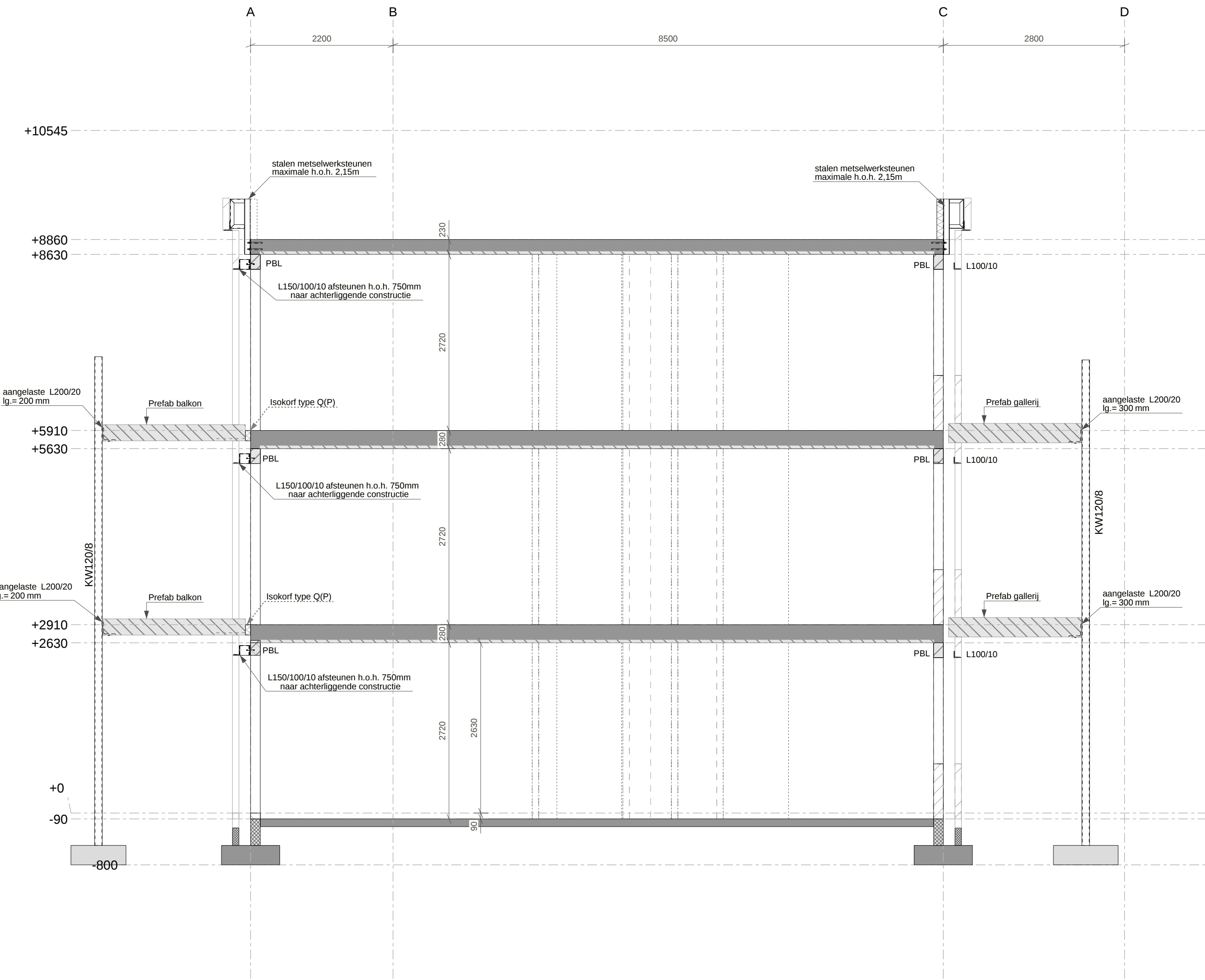
dsn II - II, 1:50
