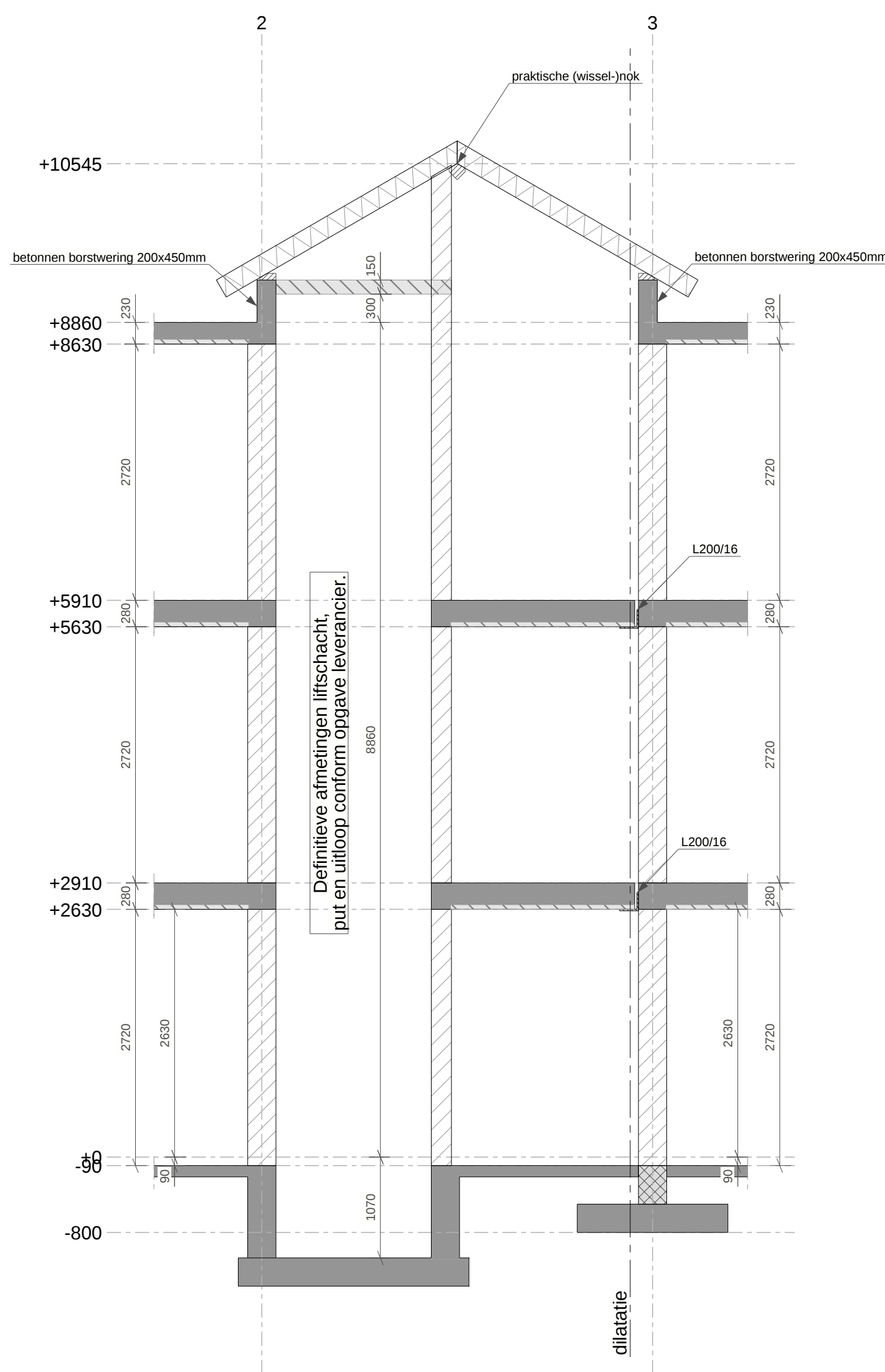
dsn III - III, 1:50
