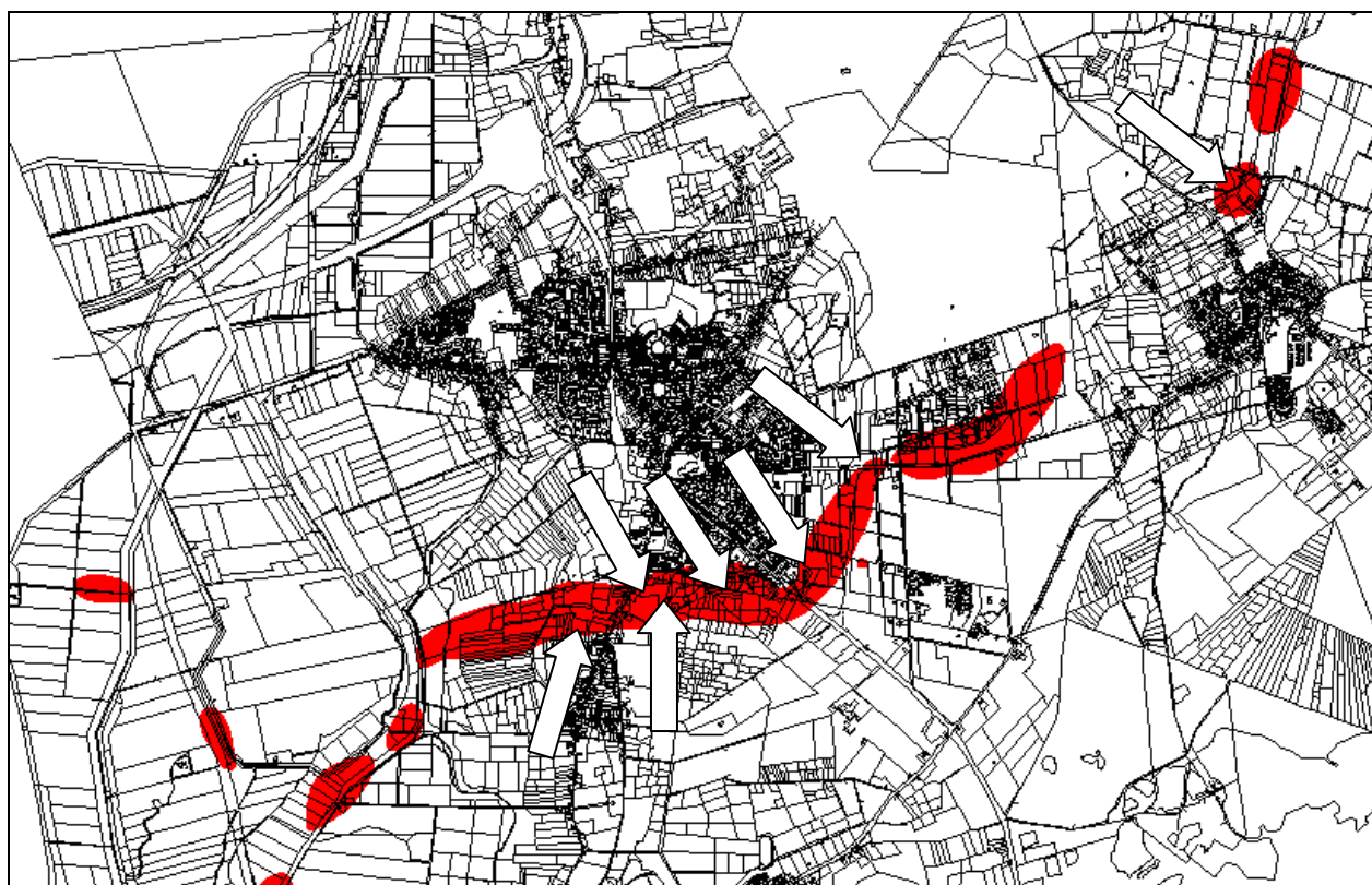
Figuur 14: Geografische ligging PR 10^{-6} contour (pijl geeft contouren met knelpunten aan)
