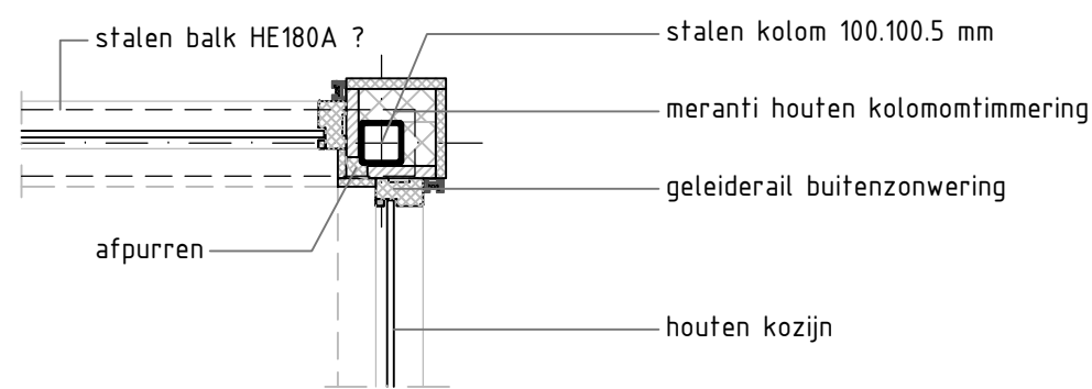
doorsnede G
