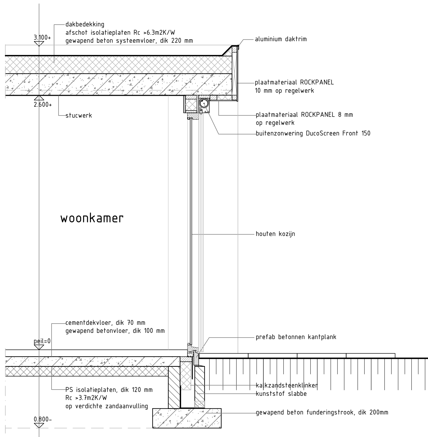
doorsnede E
