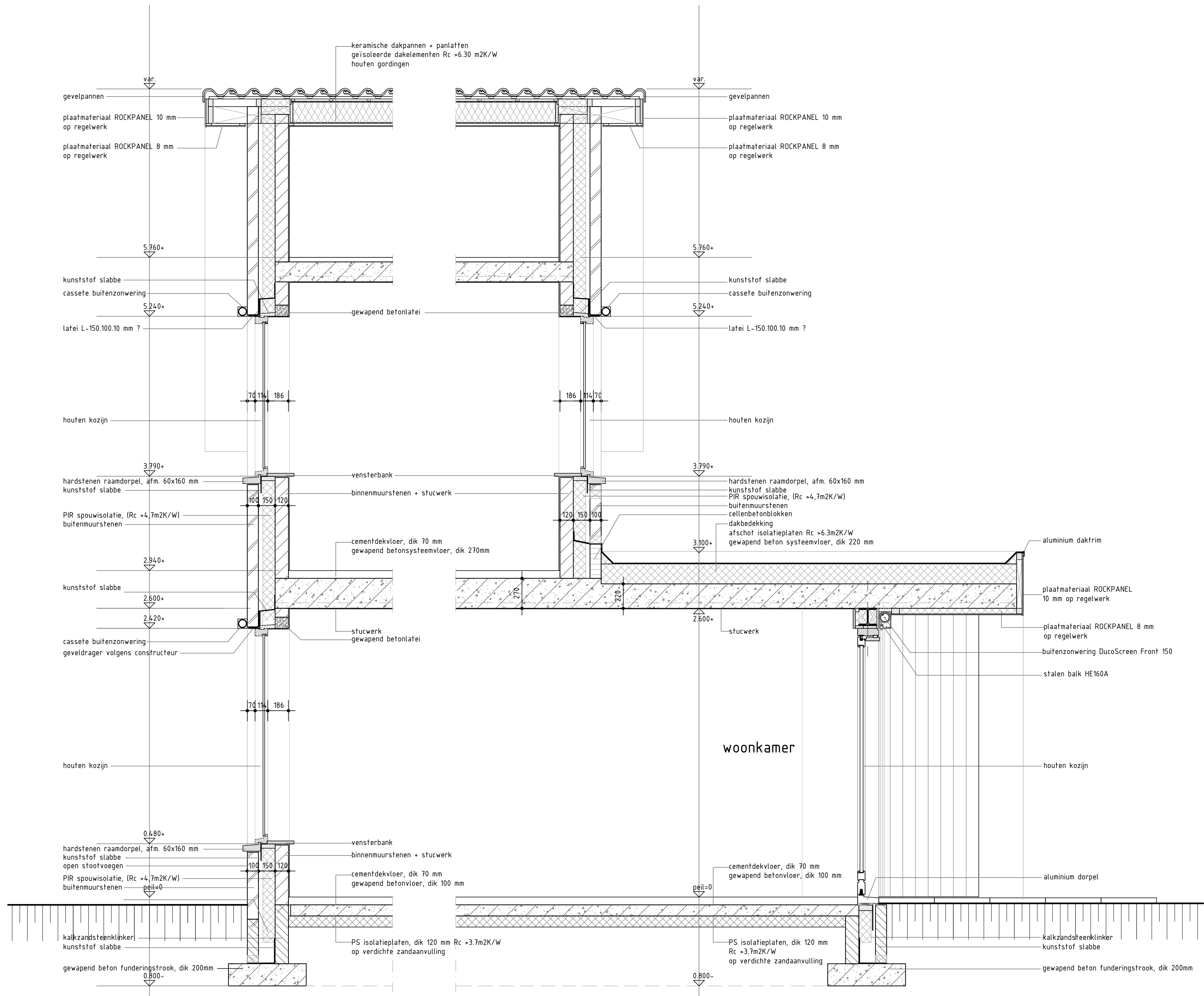
doorsnede C
