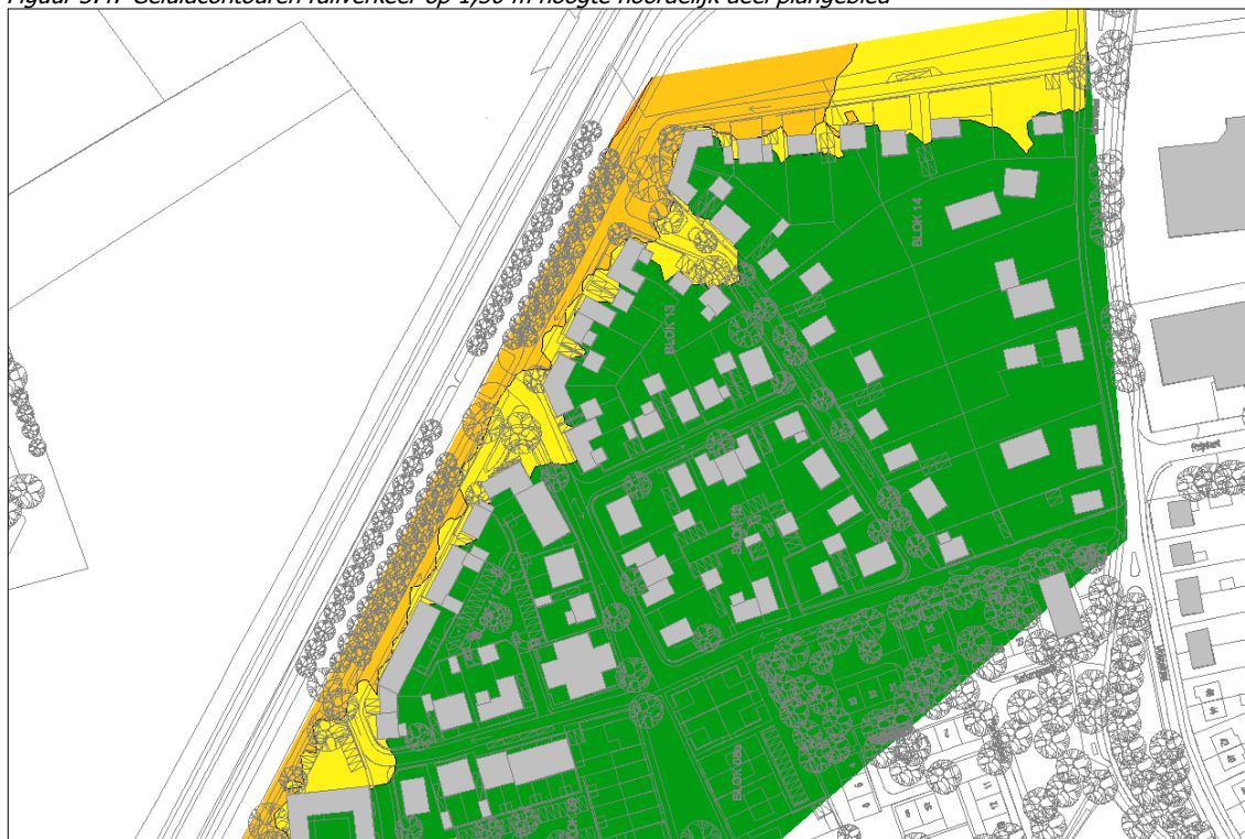
Figuur 3.4: Geluidcontouren railverkeer op 1,50 m hoogte noordelijk deel plangebied
