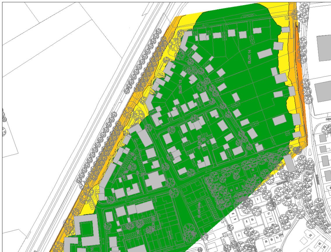
Figuur 3.6: Geluidcontouren wegverkeer op 4,50 m hoogte inclusief aftrek artikel 110g Wgh noordelijk deel plangebied
