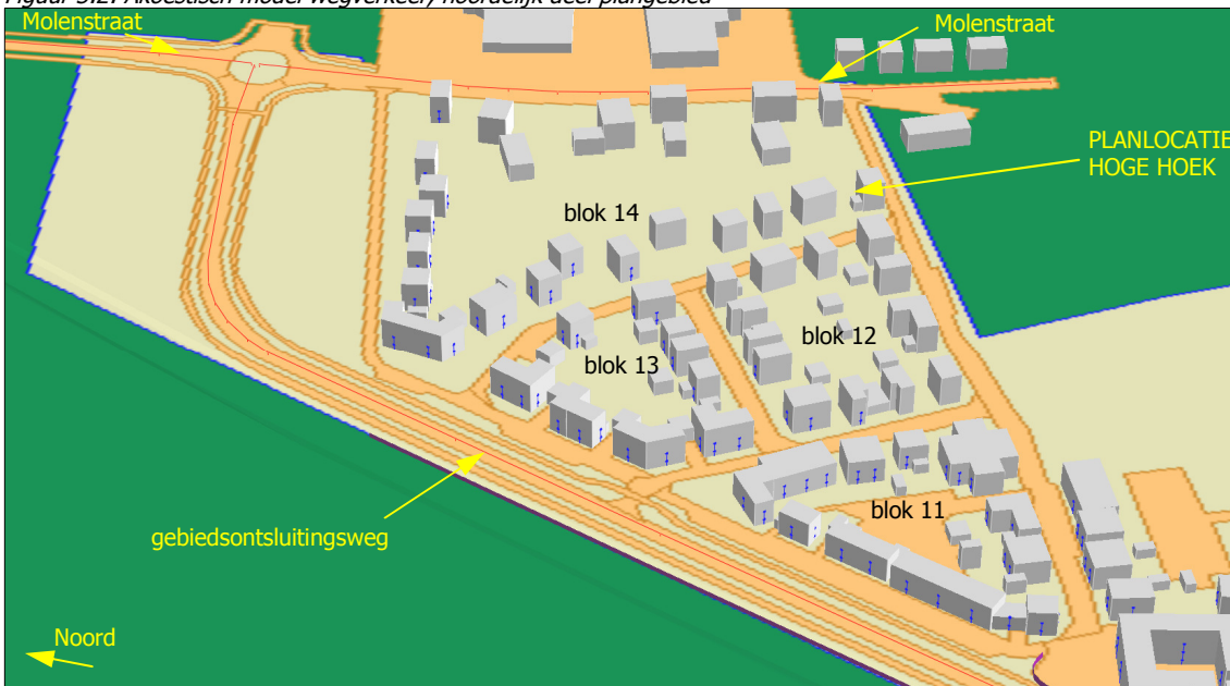
Figuur 3.2: Akoestisch model wegverkeer, noordelijk deel plangebied
