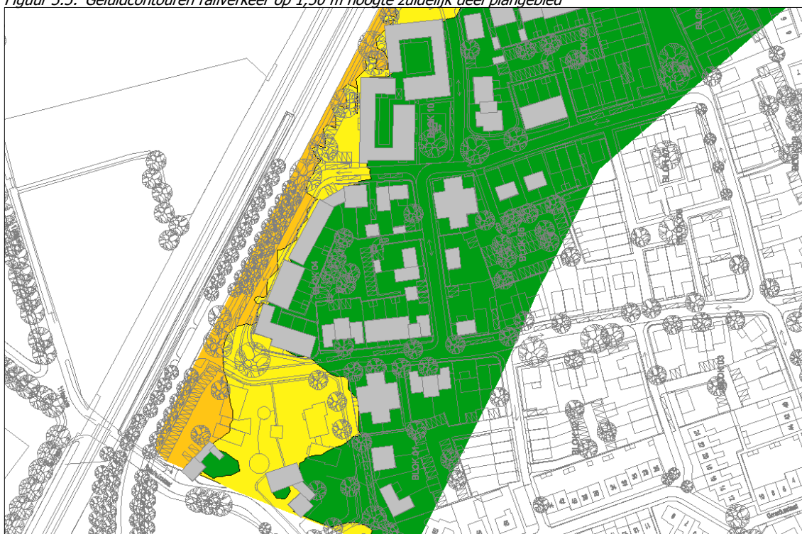
Figuur 3.5: Geluidcontouren railverkeer op 1,50 m hoogte zuidelijk deel plangebied
