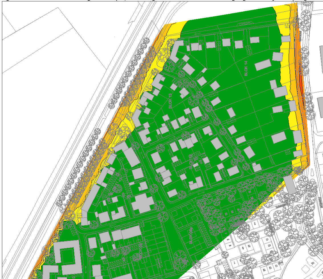
Figuur 3.4: Geluidcontouren wegverkeer op 1,50 m hoogte inclusief aftrek artikel 110g Wgh noordelijk deel plangebied
