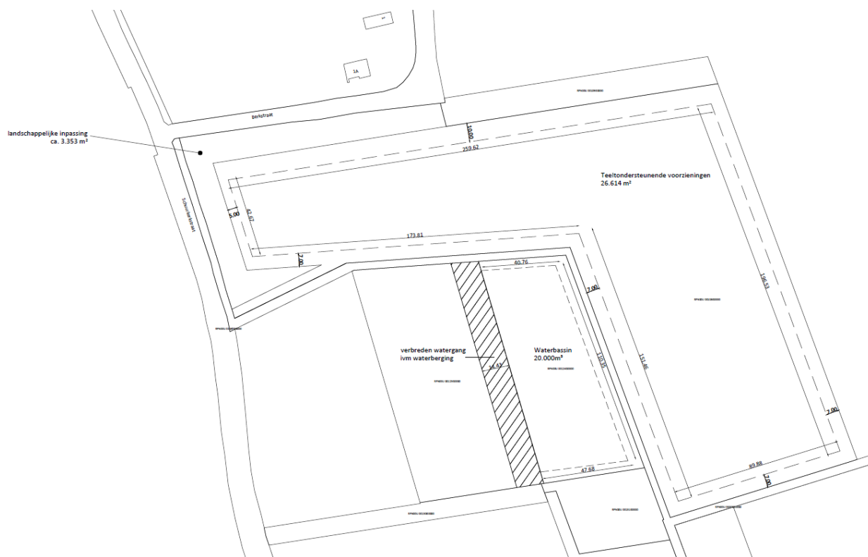
Figuur 20: nieuwe situatie reservering verbrede B-watergang
