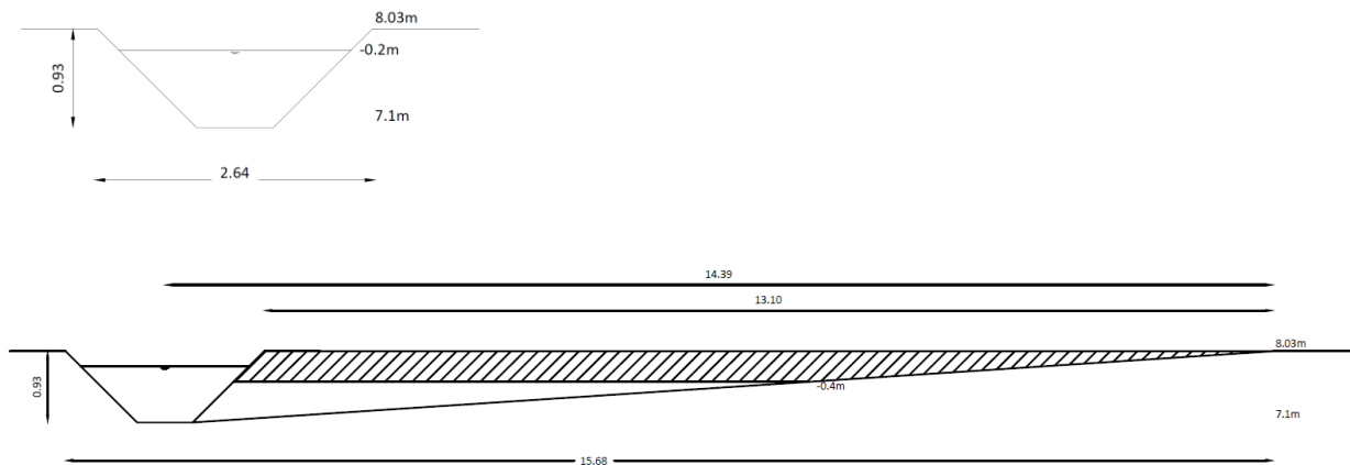
Figuur 19: bestaande en nieuwe situatie principe profiel B-watergang
