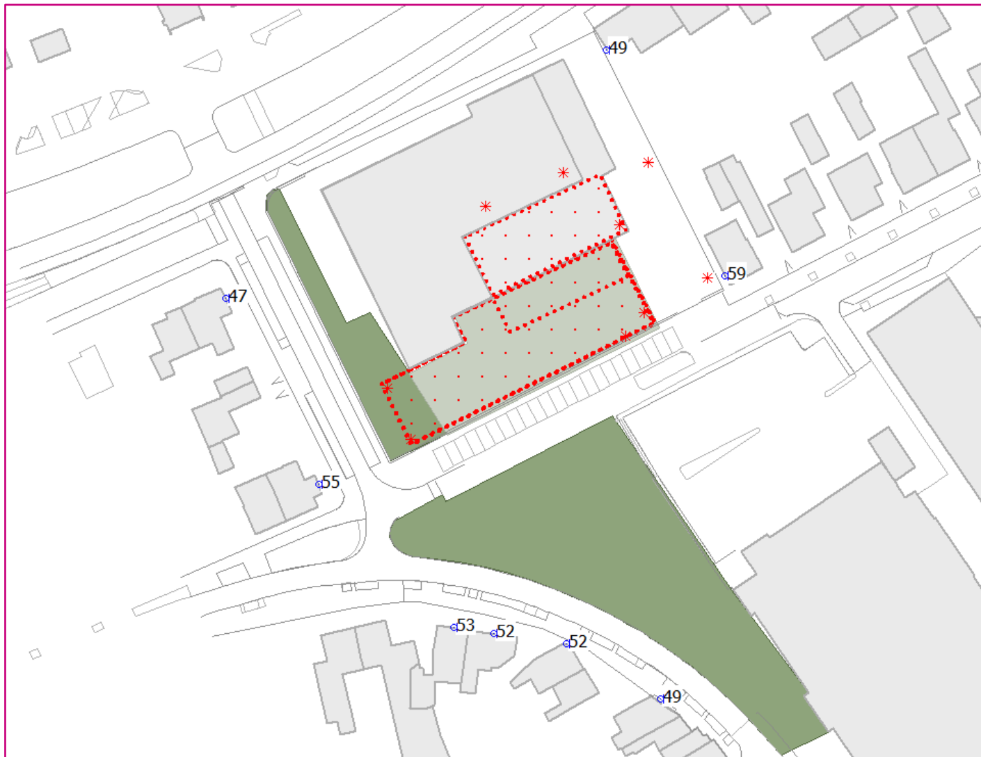
Figuur 5.1 Rekenresultaten langtijdgemiddeld beoordelingsniveau, h_o = 5 m
