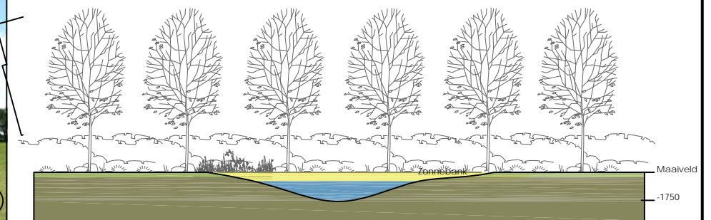
Doorsnede B-B paddenploel
