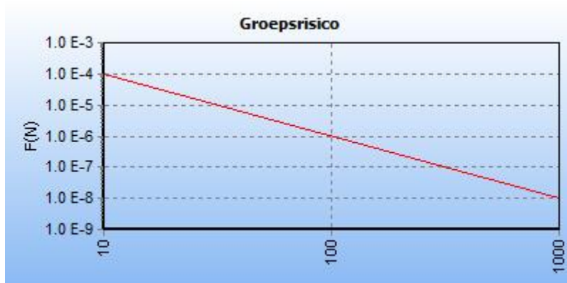
5.7 Figuur 5.7 FN curve voor 6270_leiding-Z-522-14-deel-1 van N.V. Nederlandse Gasunie voor de kilometer tussen stationing 0.00 en stationing 240.00
