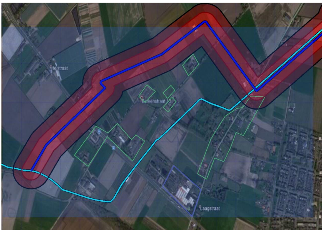
3.4 Figuur 3.4 Plaatsgebonden risico voor 6270_leiding-Z-521-08-deel-1 van N.V. Nederlandse Gasunie
