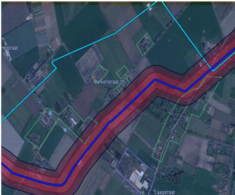
3.2 Figuur 3.2 Plaatsgebonden risico voor 6270_leiding-Z-521-01-deel-1 van N.V. Nederlandse Gasunie
