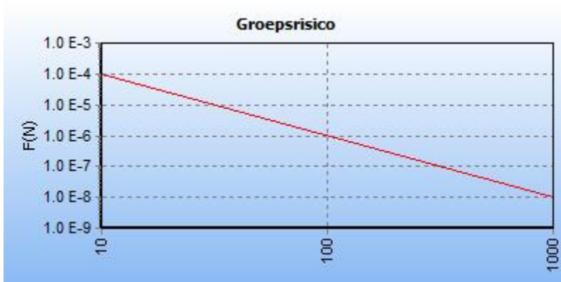
5.5 Figuur 5.5 FN curve voor 6270_leiding-Z-522-01-deel-1 van N.V. Nederlandse Gasunie voor de kilometer tussen stationing 1290.00 en stationing 2290.00
