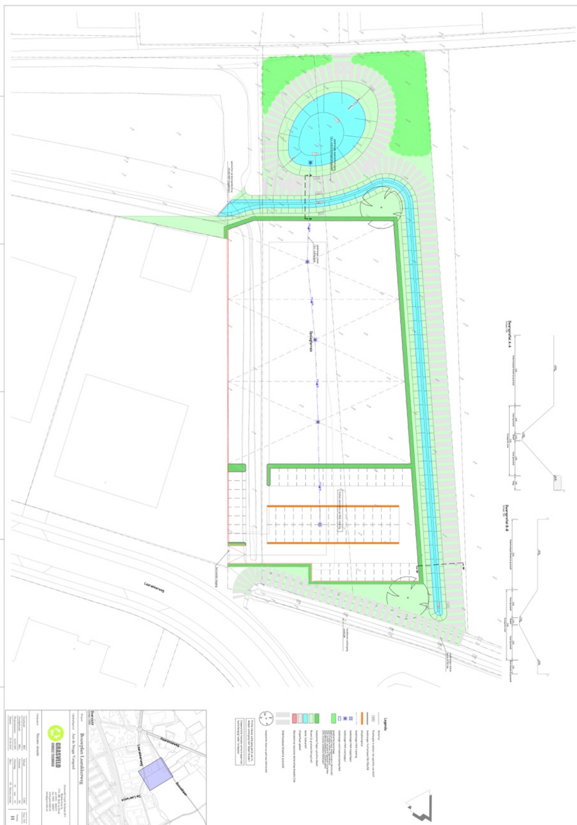
Afbeelding 2: geplande inrichting
