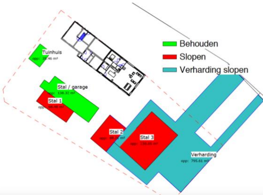
Figuur 6: illustratie van de te slopen en te behouden gebouwen en op te breken verharding (mestsleuf)
