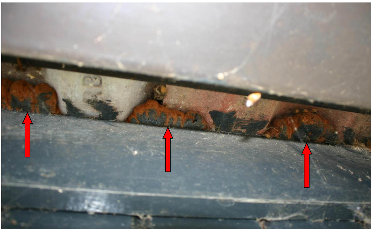
Figuur 5. Onderaanzicht van het dak van het schuurtje. De 'golven' zijn allemaal opgevuld (rode pijlen).
