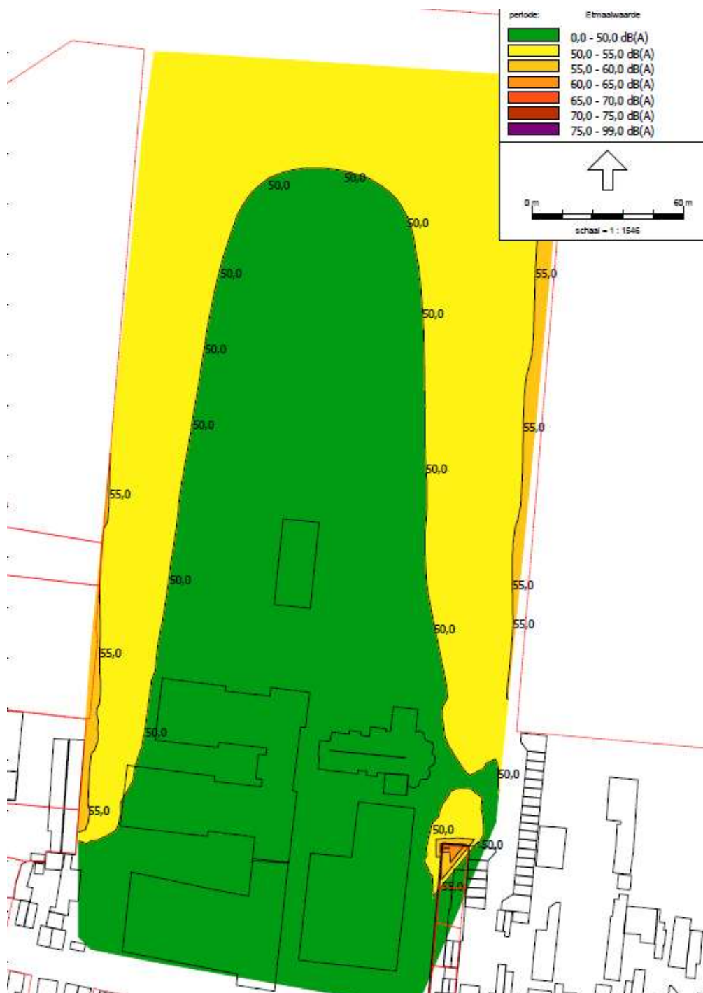
Figuur 4.13: De binnen het plan optredende gecumuleerde langtijdgemiddelde beoordelingsniveaus
