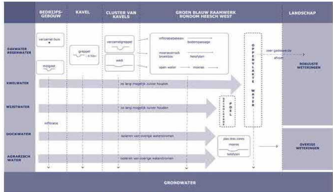
Visie schema watersysteem van kavel tot landschap
