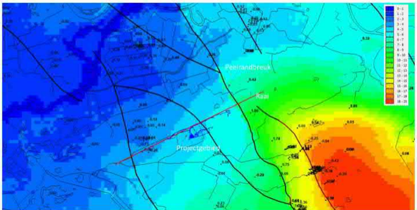
Figuur B1.1 Berekende freatische grondwaterstand en de afwijkingen in modellaag 4.
