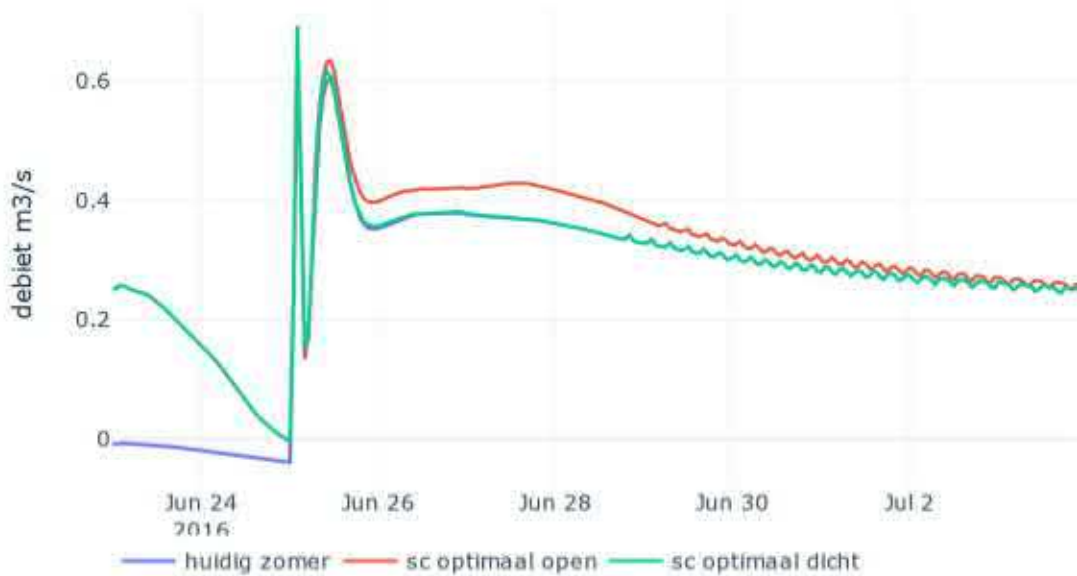
Figuur 4-18: Zuidelijke flux voor huidig en optimaal scenario in de zomer.
