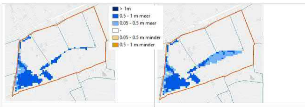
figuur 4-3: overstromingspatroon winter T=100 scenario 1 (links) en scenario 3 (rechts)
