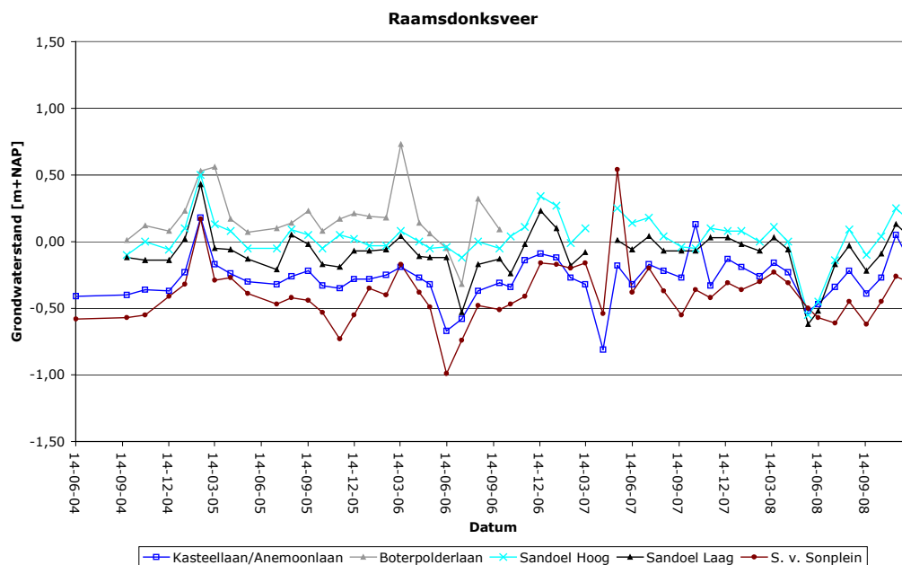
afbeelding 4.2. Grondwaterstandsverloop t.o.v. NAP
