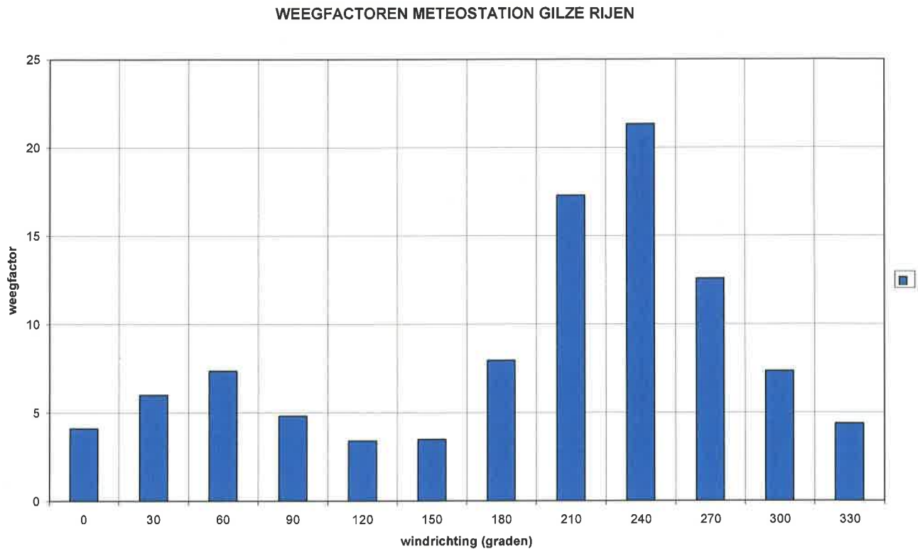
Figuur 13 Weegfactoren voor meteostation Gilze Rijen.
