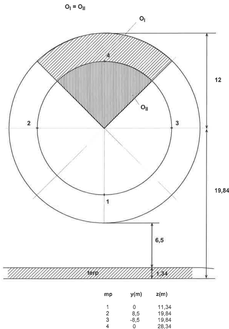
Figuur 4 Ligging van de meetposities binnen het wiekoppervlak van de molen.
