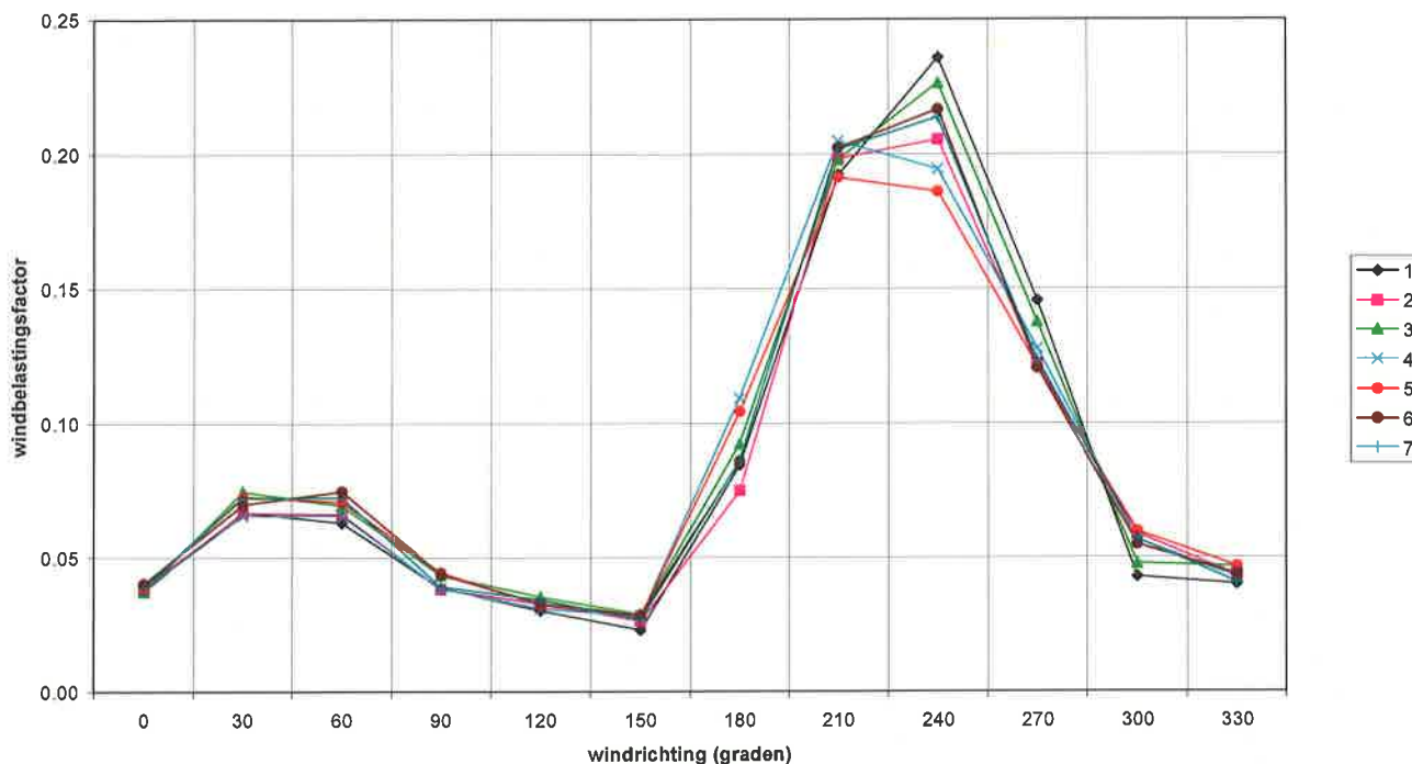
Figuur 18 Gewogen windbelastingen over het wiekoppervlak.
