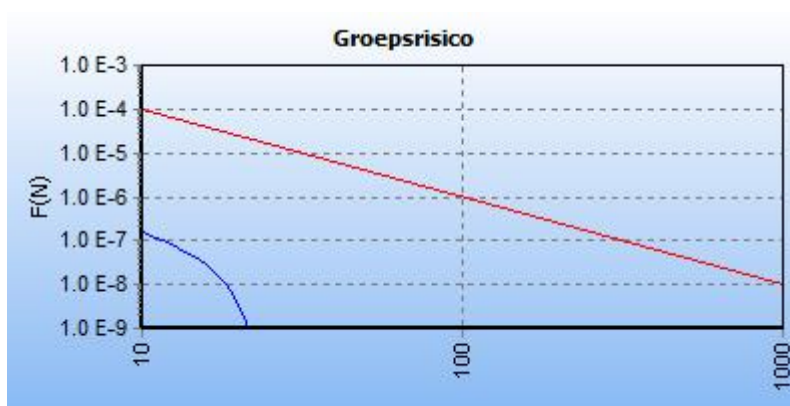
Afbeelding 6 fN-curve buisleiding Z-519-01-deel-1, huidige situatie
