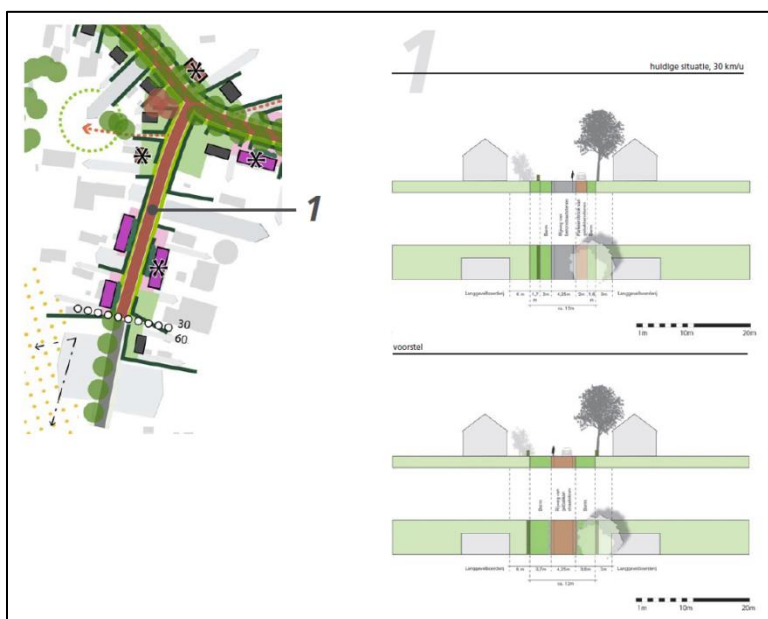
Afbeelding 10: Beeldkwaliteitsplan Groenstraat Wintelre
