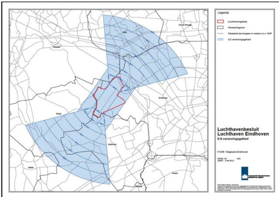
Kaart obstakelbeheergebied instrument landing systeem
