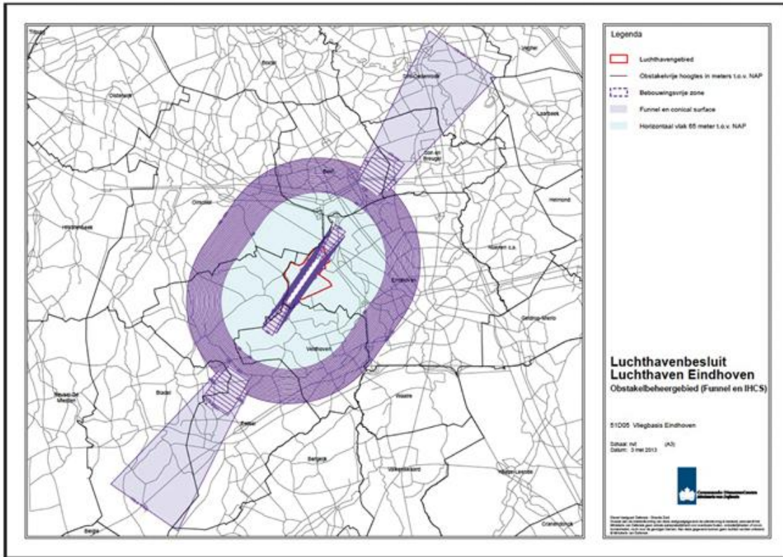
Kaart obstakelbeheergebied vliegfunnel en IHCS
