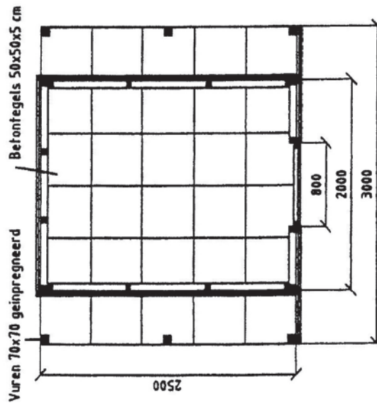
Plattegrond
