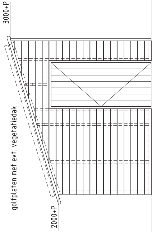
VOORGEVEL
