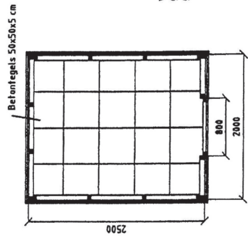
Plattegrond
