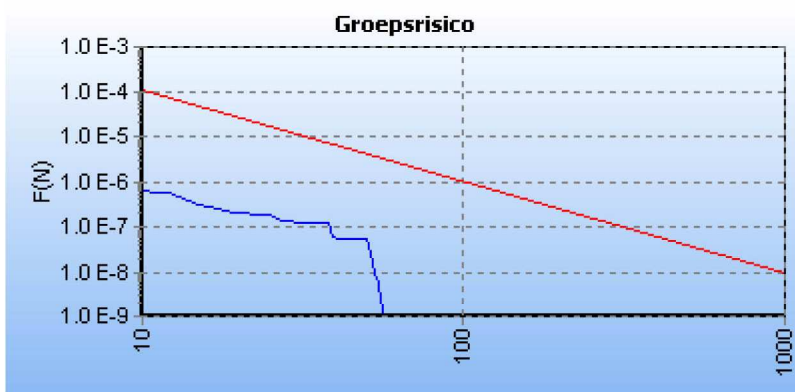
5.1 Figuur 5.1 FN curve voor {C8314B50-44B0-485C-8BEB-0AFAA534EF9E}_000178 van Nederlandse Aardolie Maatschappij BV voor de kilometer tussen stationing 2210.00 en stationing 3210.00
