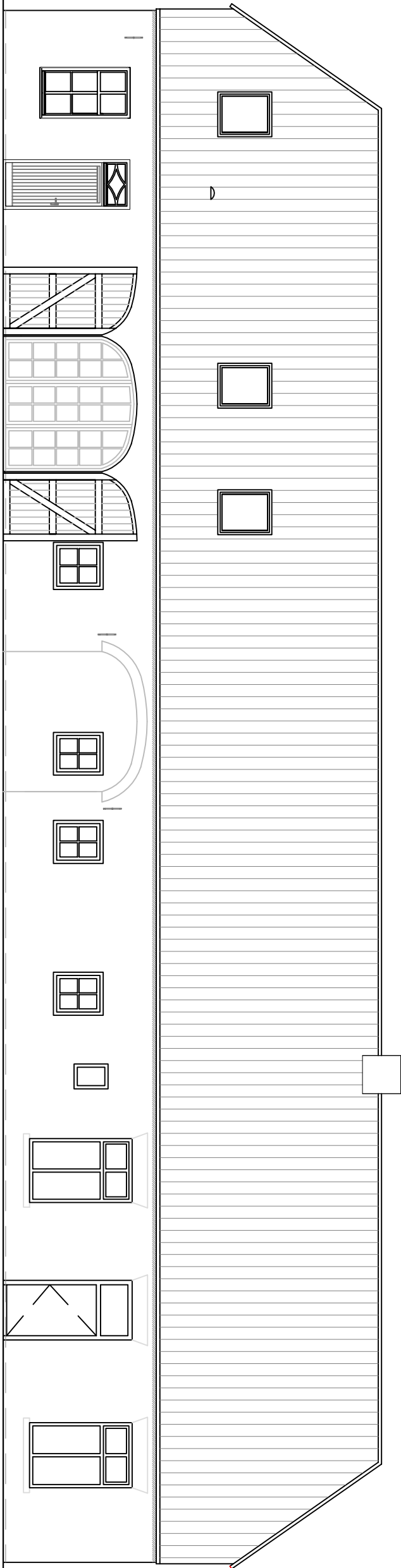
HUIDIGE VOORGEVEL
