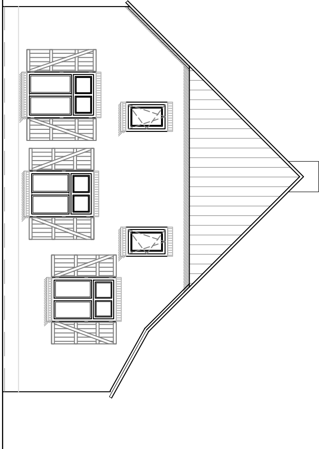
NIEUWE RECHTER ZIJGEVEL
