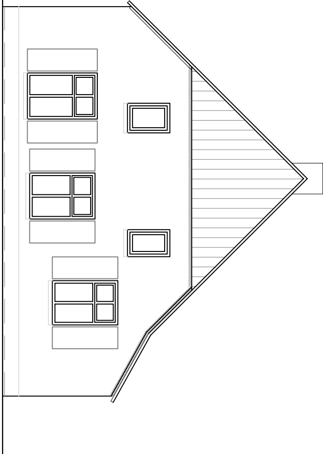
HUIDIGE RECHTER ZIJGEVEL
