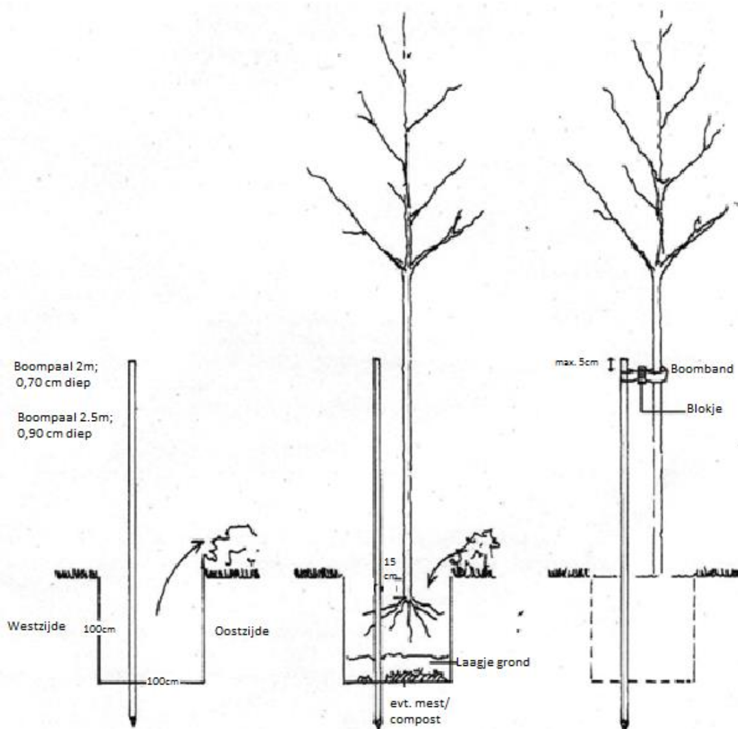
Afbeelding 4: Plantinstructies bomen
