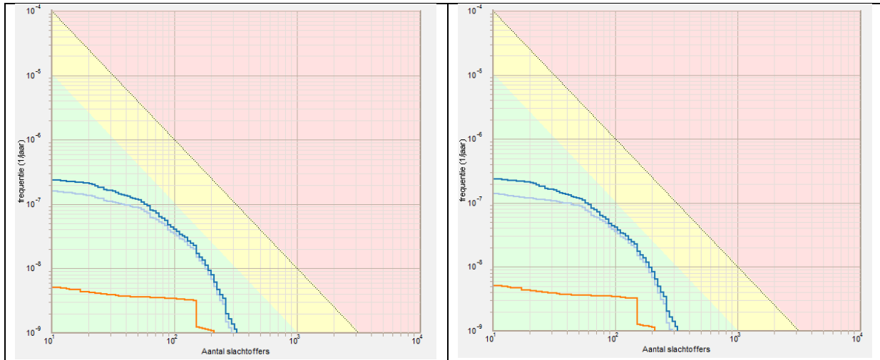
Figuur 4.2 Gesommeerd groepsrisico als gevolg van transport per spoor in huidige (links) en toekomstige situatie
