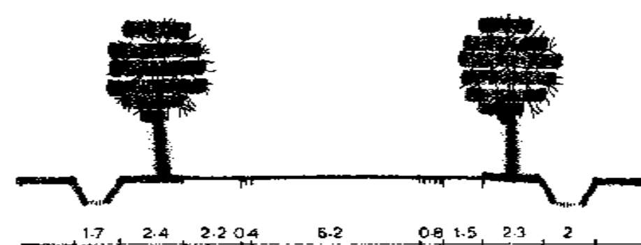
PROFIEL 7
