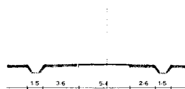
PROFIEL 3
