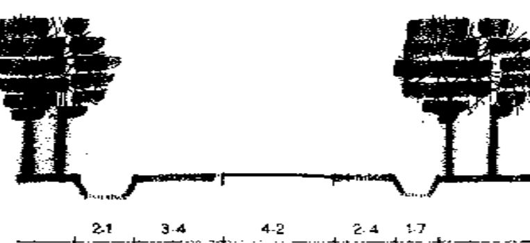
PROFIEL 9
