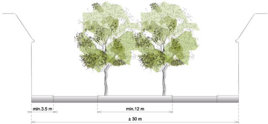
boulevard profiel
