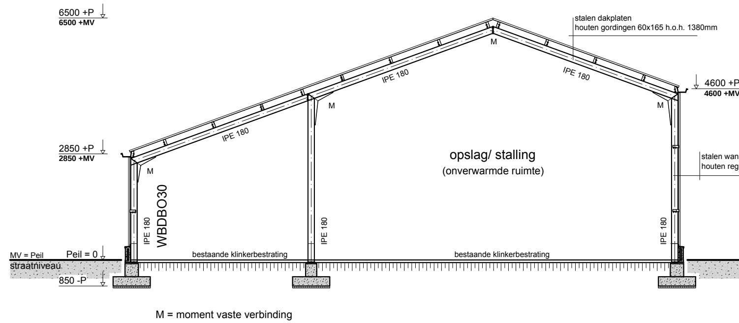
Doorsnede A-A
