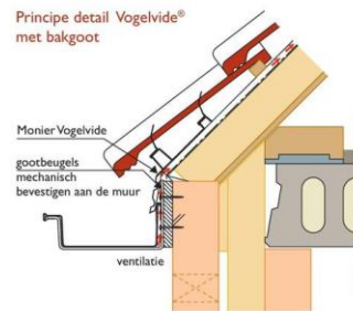
Principe detail Vogelvide® met zinken goot
